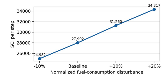
(그림 1) 정규화 연료소비 교란에 따른 Double DQN SCI/step
