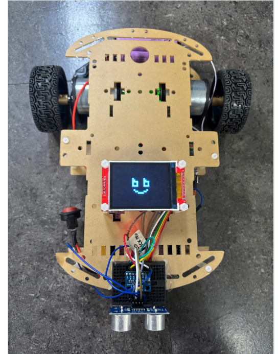
실제 제작한 RC카 · IMU 연동 LCD 화면 · 팀 발표자료 사진
