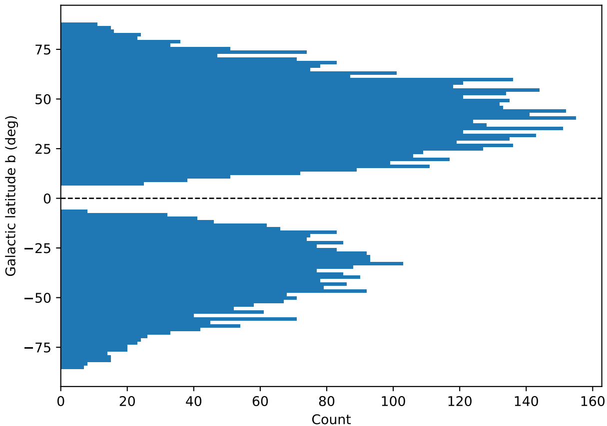
Distribution of Galactic latitude
