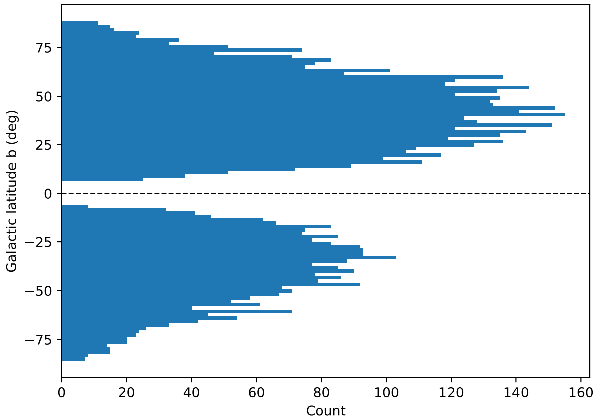
Distribution of Galactic latitude
