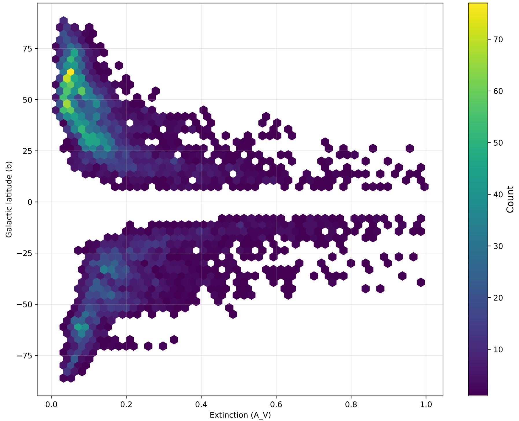
Extinction vs Galactic latitude
