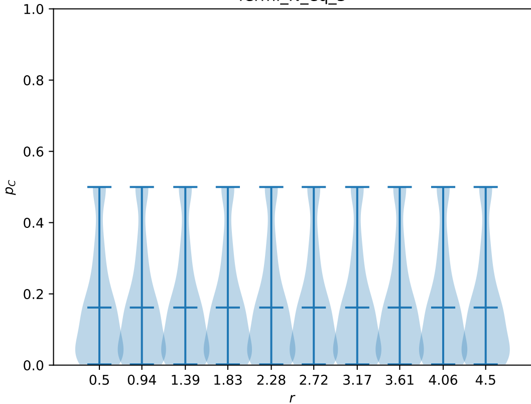
fermi_N_eq_3
