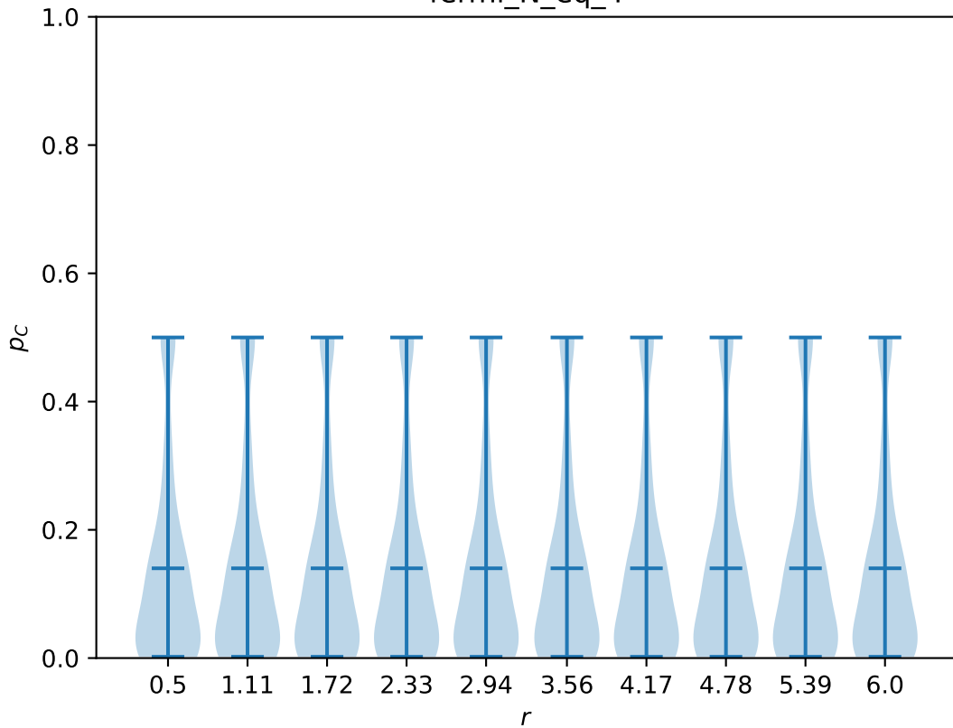
fermi_N_eq_4
