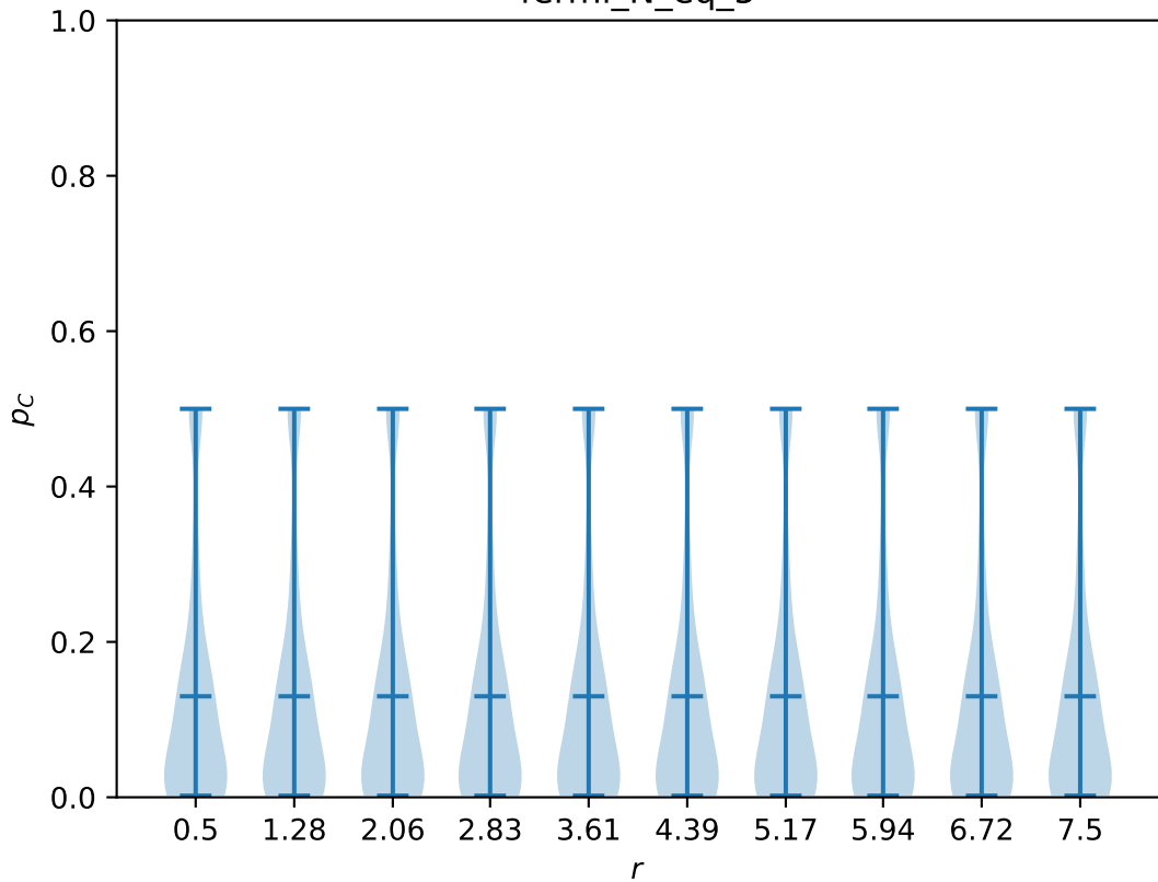
fermi_N_eq_5
