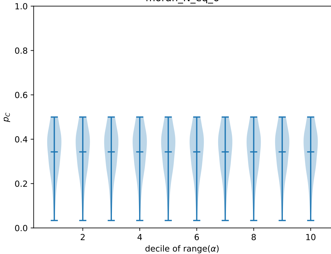
moran_N_eq_6
