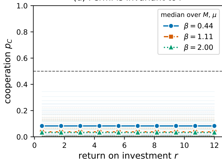
(d) Fermi is invariant to r
