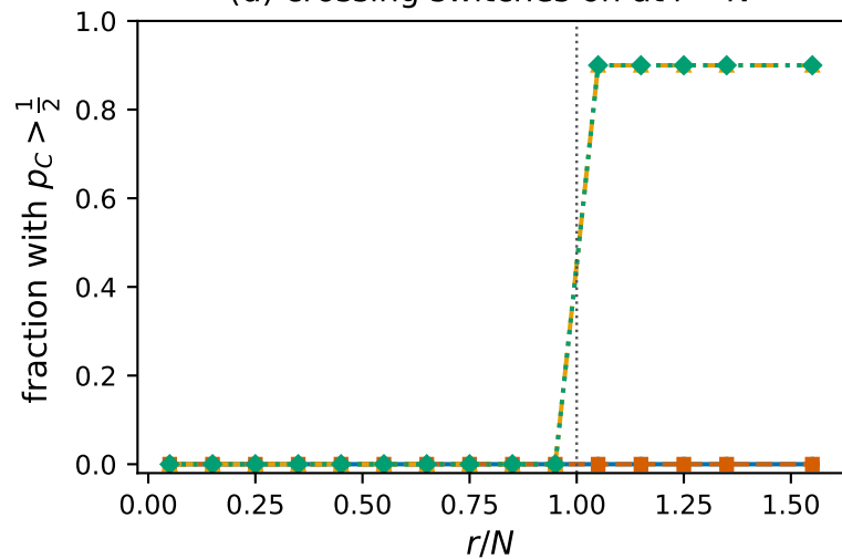
(d) crossing switches on at r = N
