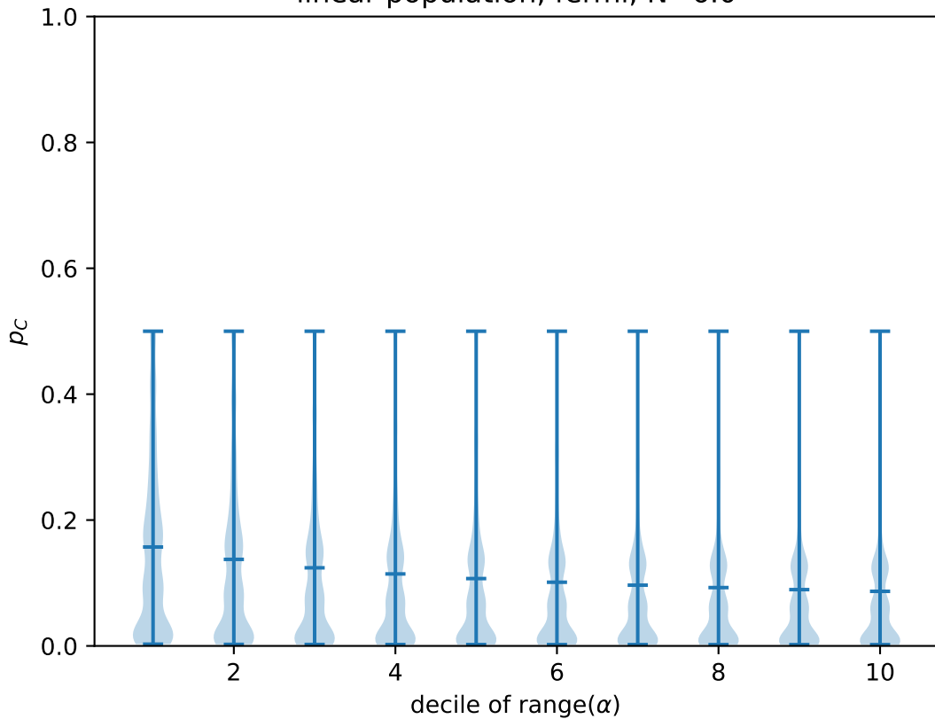
linear population, fermi, N=6.0
