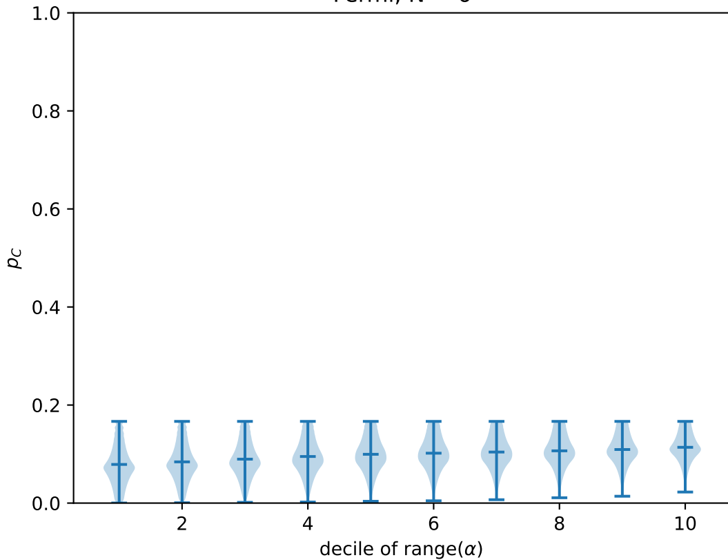
Fermi, N = 6
