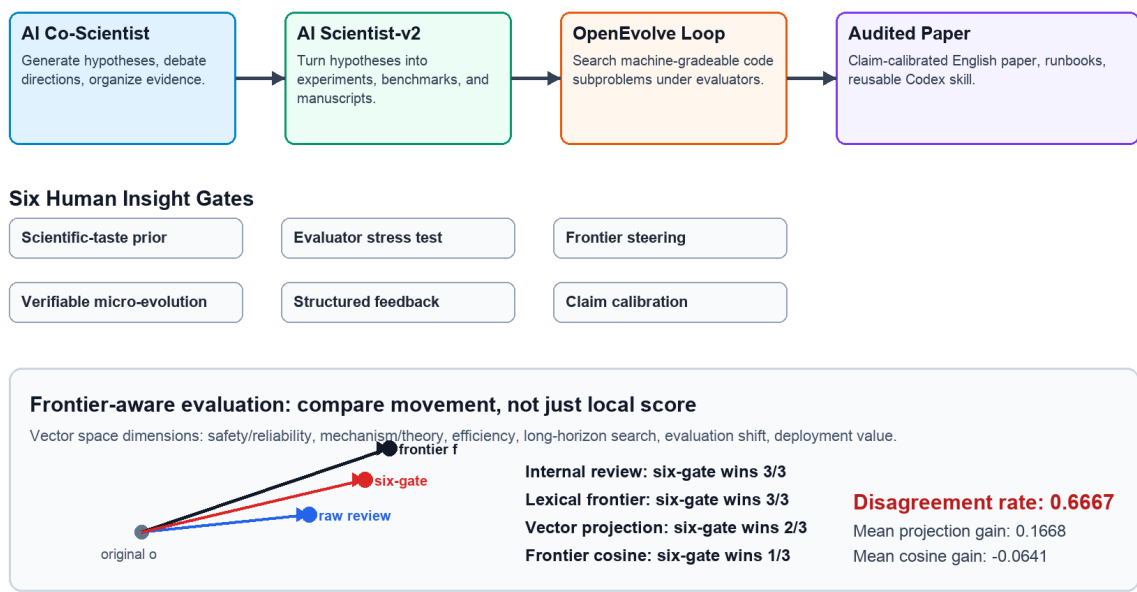
图 1. Co-Pilot AI Scientist v3 结合 AI Co-Scientist 式假设前沿、AI Scientist-v2 式实验与论文生产、OpenEvolve 式微搜索，以及六类人类洞察门控。下半部分展示为什么前沿感知评估需要向量移动和指标分歧，而不是单一短期分数。
