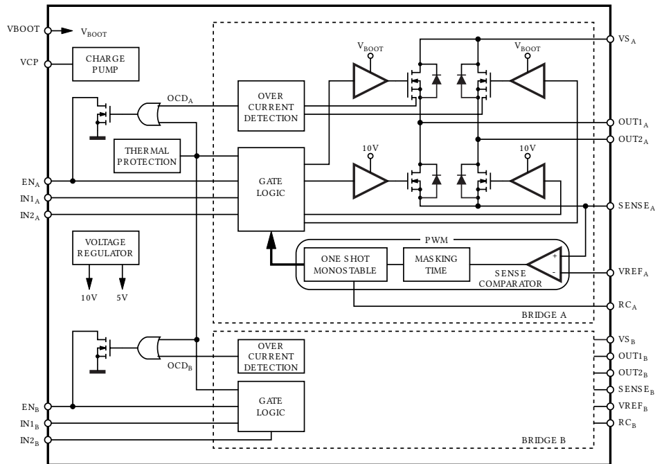
Figure 8 - Schéma bloc du circuit du pont-H L6207N [4]
