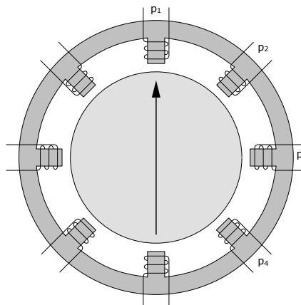
Figure 9 - Schéma de principe du moteur pas-à-pas.
