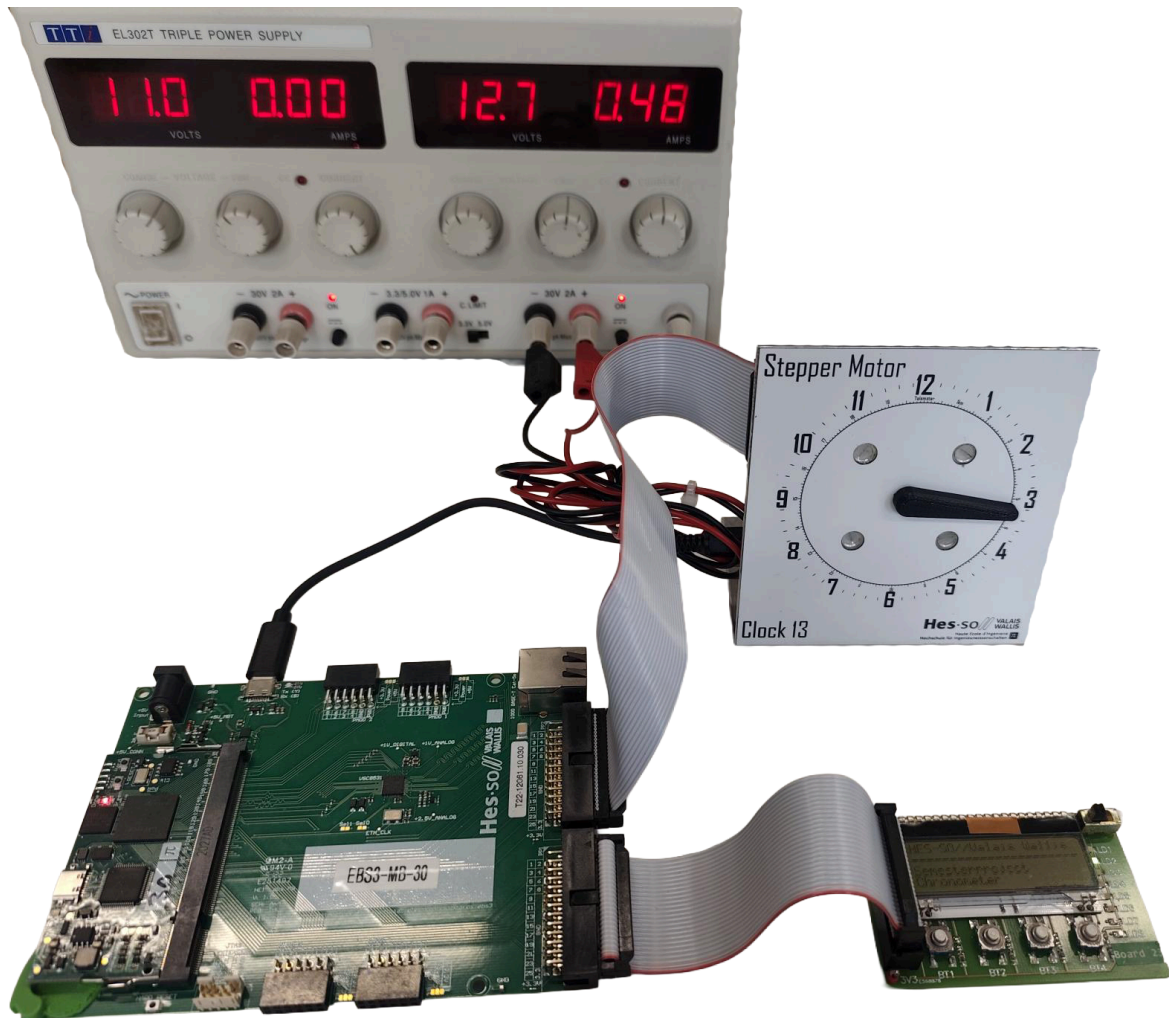
Figure 1 - Équipement du chrono (EBS3)
