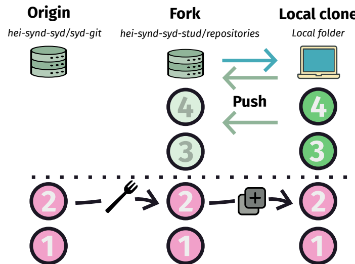
Abbildung 18 - Push auf das Remote-Repository
