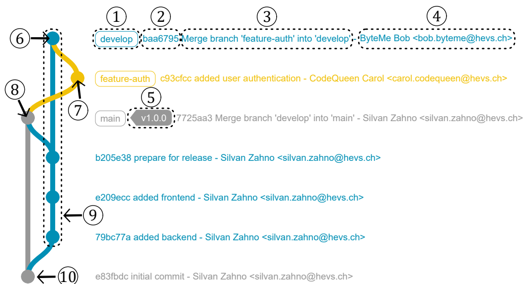
Abbildung 30 - Beispiel eines Gitgraphen
