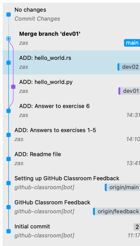
Figure 21 - Statut après la fusion des branches dev01 et dev02 du repo
