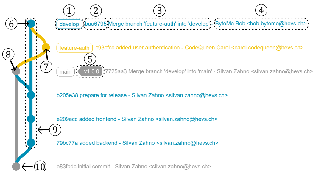
Figure 23 - Exemple d'une gitgraphe
