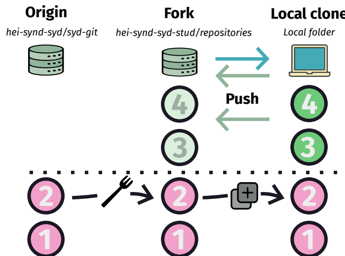
Figure 11 - Push sur le dépôt distant
