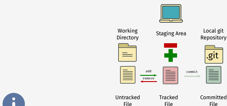
Figure 8 - Types d'opérations locales de Git
