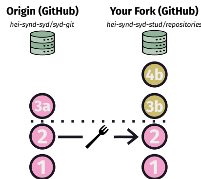
Abbildung 9 - Fork des Vorlagen-Repositories
