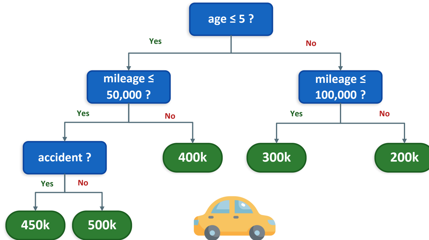
Decision Tree สำหรับประมาณราคารถยนต์มือสอง
