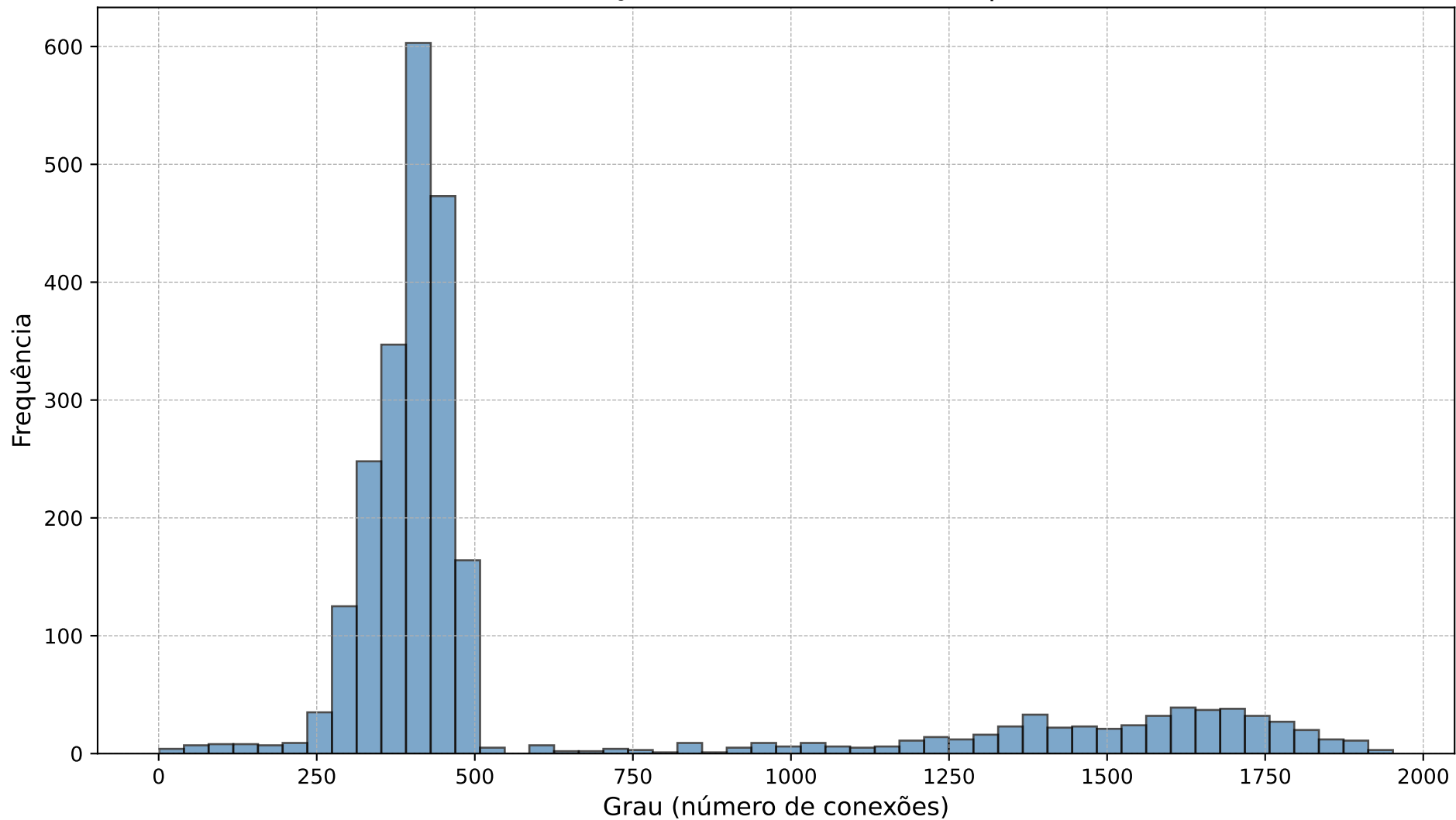
Distribuição de Graus - Grafo Completo
