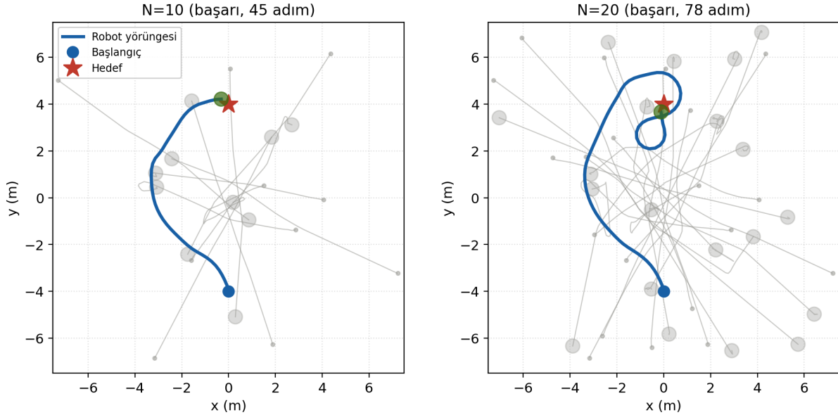
Şekil 5. Şampiyon (v30) gerçek yörüngeleri (paper_challenging, robot 1.0 m/s). Mavi: robot yörüngesi; gri: yayalar (yol + son konum); kırmızı yıldız: hedef. Robot her iki yoğunlukta da kavisli kaçınma yapar; N=20'de güzergâh belirgin biçimde uzar (gerçek kaçınma, beeline değil).
