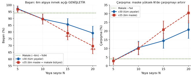
Şekil 7. Algı-menzili ablasyonu (v35). v30 (tüm yayalar) ile v35 (6 m maske = makale bütçesi) ve makale (yeşil) karşılaştırması. 6 m bütçeye inmek başarıyı yüksek-N'de düşürür (sol) ve çarpışmayı artırır (sağ): algı menzili açığın nedeni değildir.
