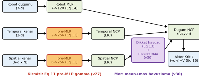
SNCP-PPO mimarisi: şampiyon (v30) sadakat eklentileri vurgulu
