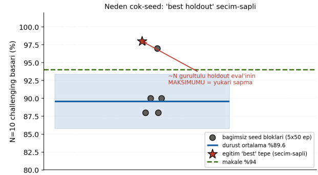
Şekil 3. N=10 ’da seçim sapması. Gri noktalar bağımsız tohum bloklarıdır; mavi bant dürüst ortalamanın %95 GA’sıdır. Kırmızı yıldız, eğitimin kaydettiği seçim-saplı “best” tepesidir. Tüm kıyaslar artık çok-tohumludur.
