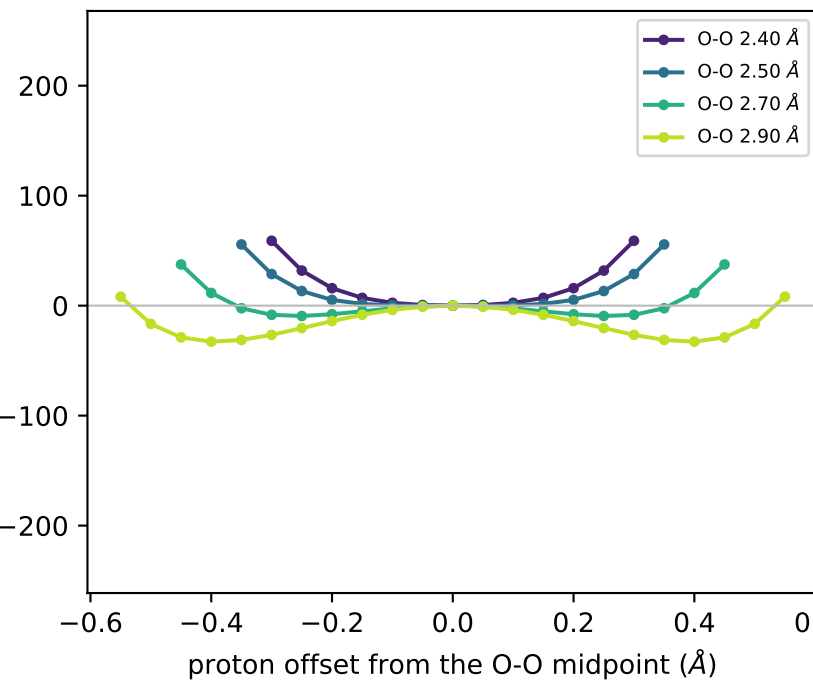
Q-Chem
