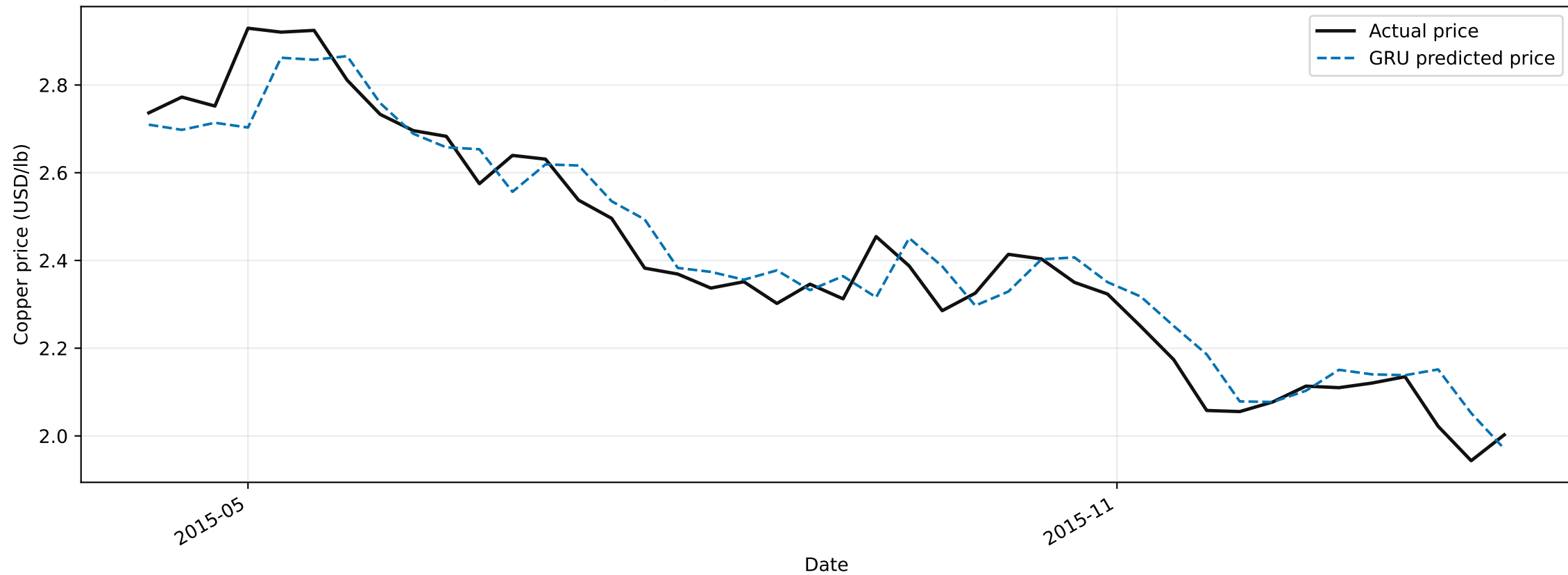
GRU prediction vs actual, h=1 Test period: 2015-04-10 to 2016-01-22
