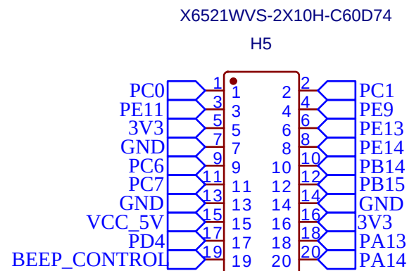
预留用户GPIO排针
