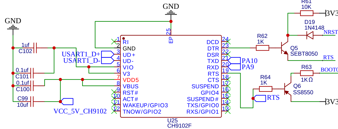
串口1一键下载电路
