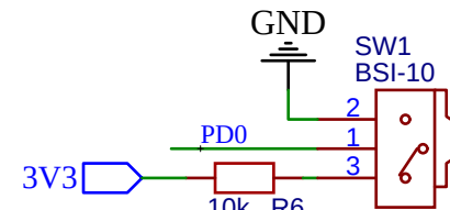
拨码开关
