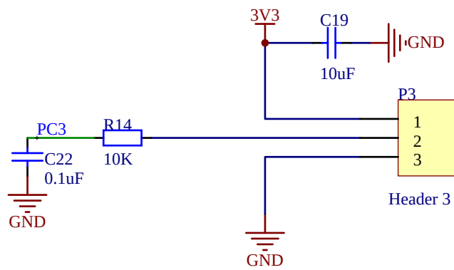
电位器（模式选择）
