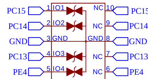
OLED接口
