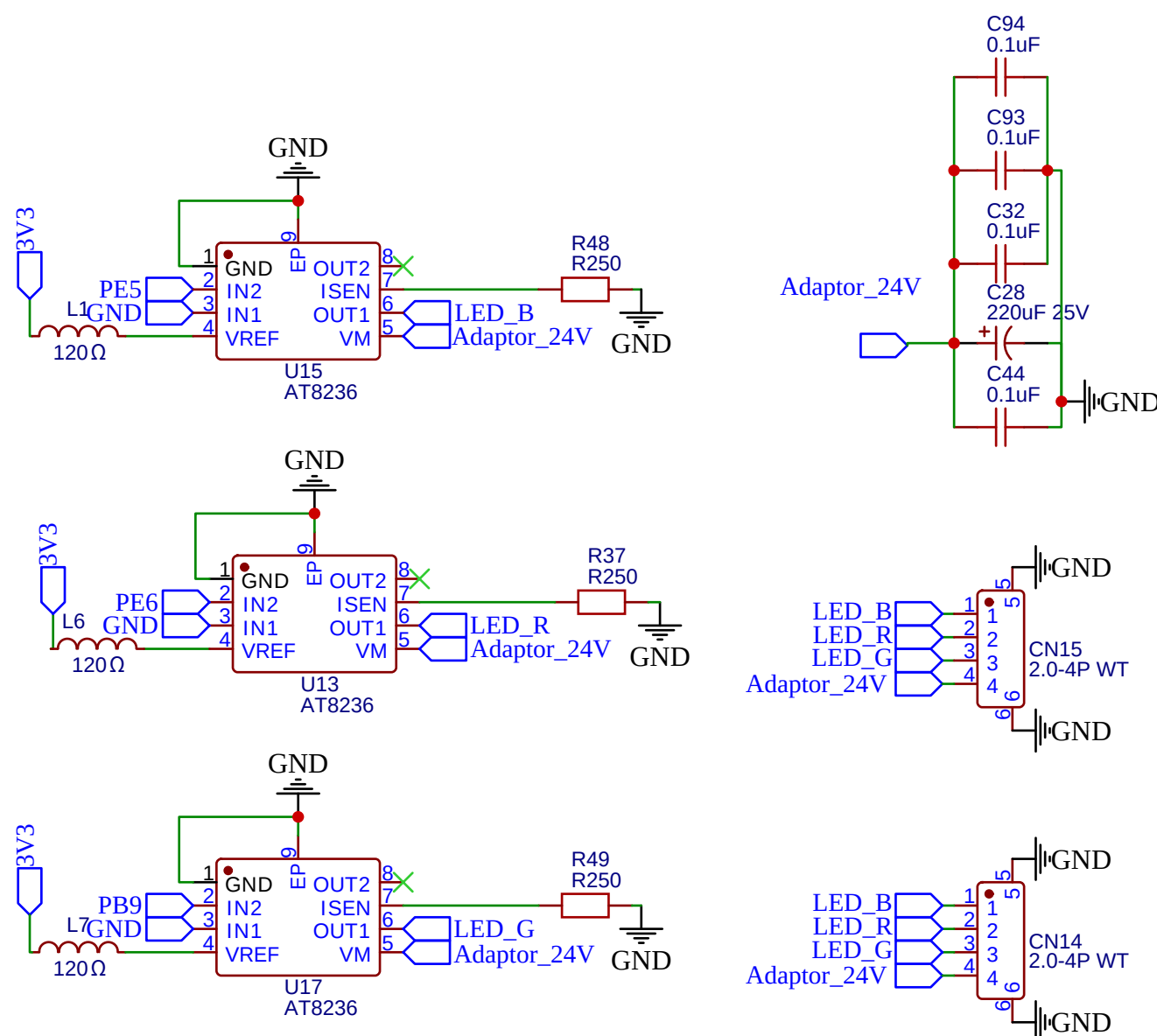
RGB_LED灯带驱动
