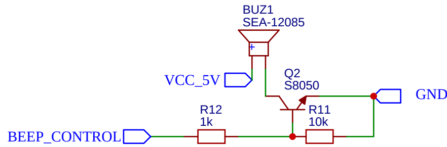
蜂鸣器
