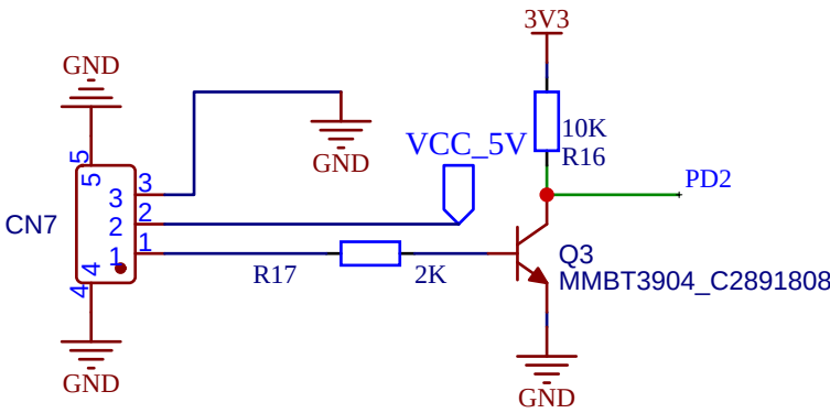
SBUS电路
