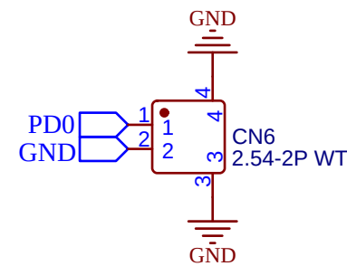
急停开关
