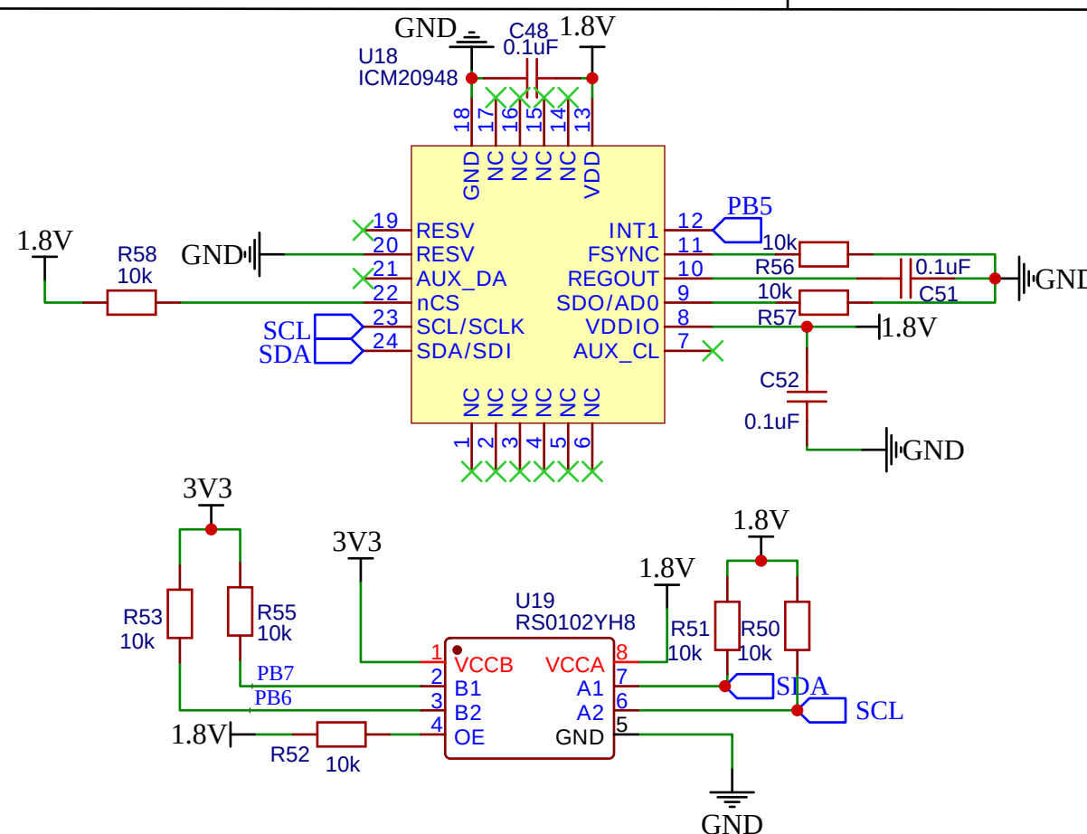
ICM20948陀螺仪
