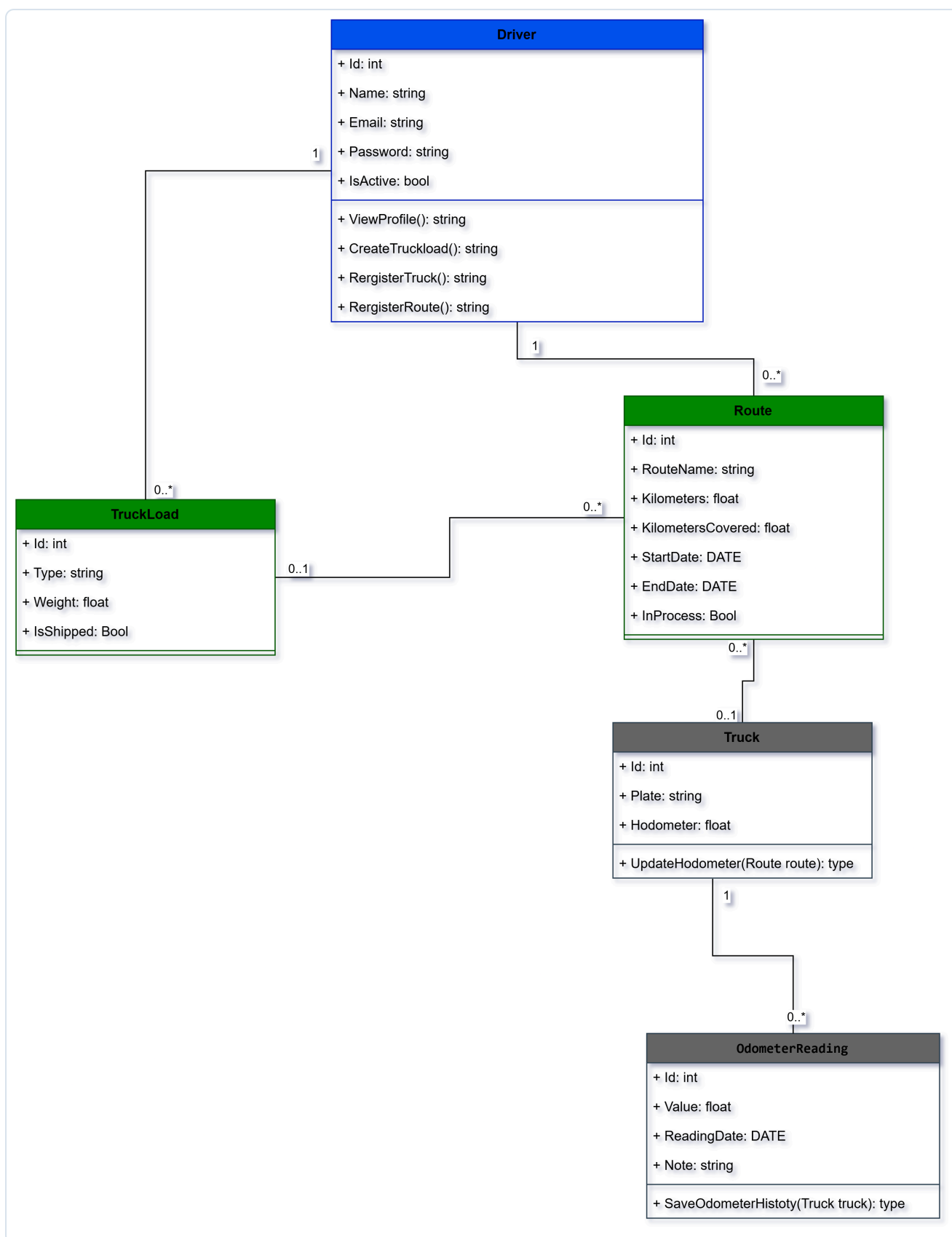
Diagrama de Classes — Estrutura de dados do Driver App
