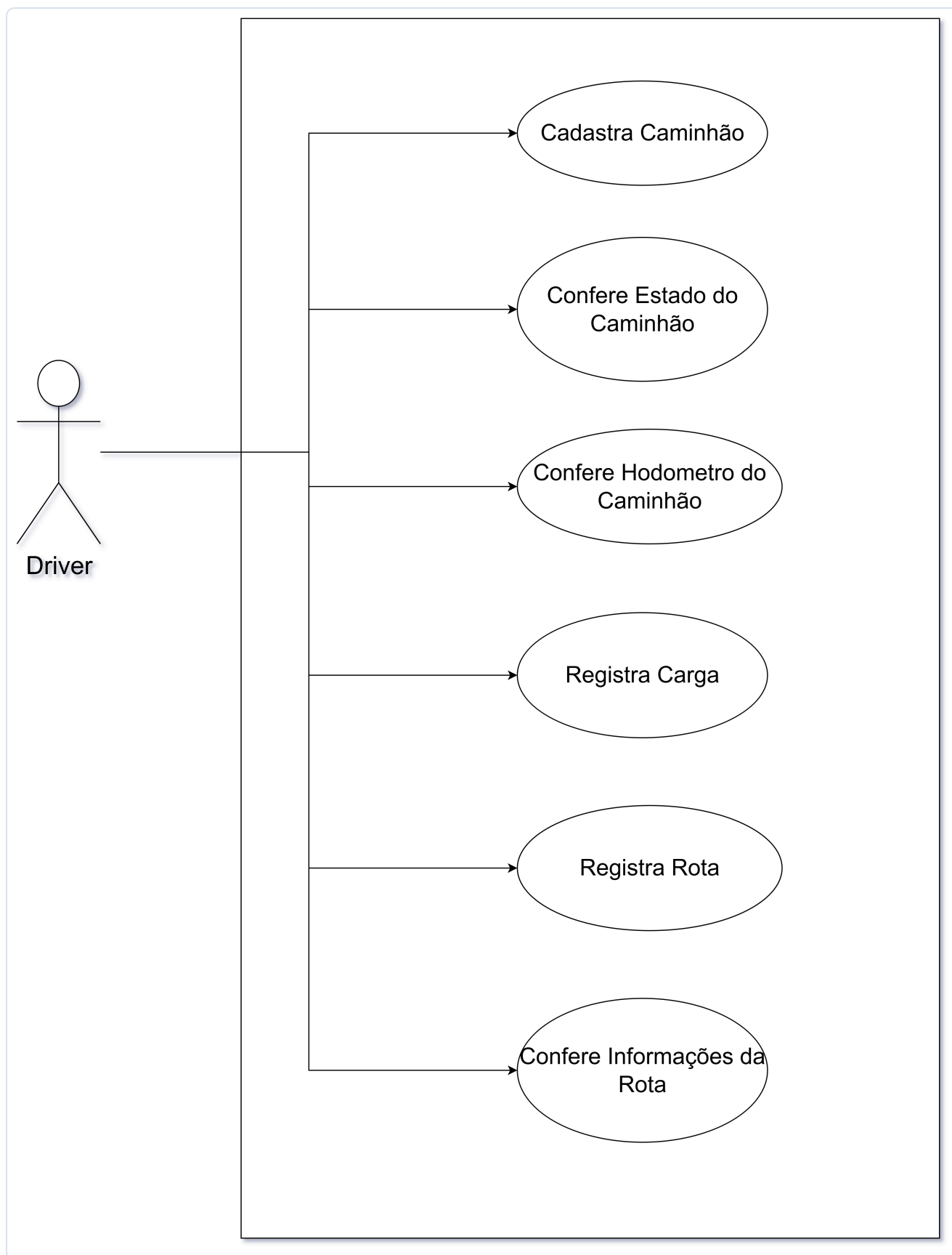
Diagrama de Caso de Uso — Ator "Driver" (Motorista)
