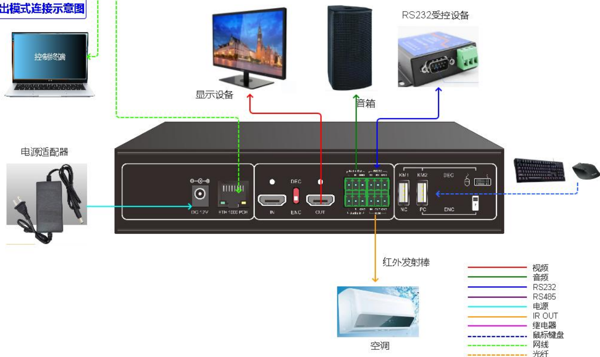
输出模式连接示意图
