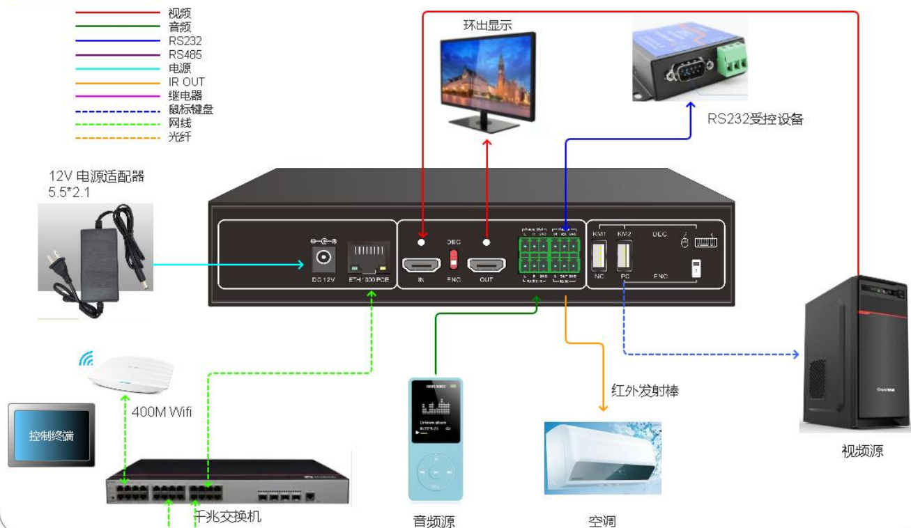
输入模式连接示意图
