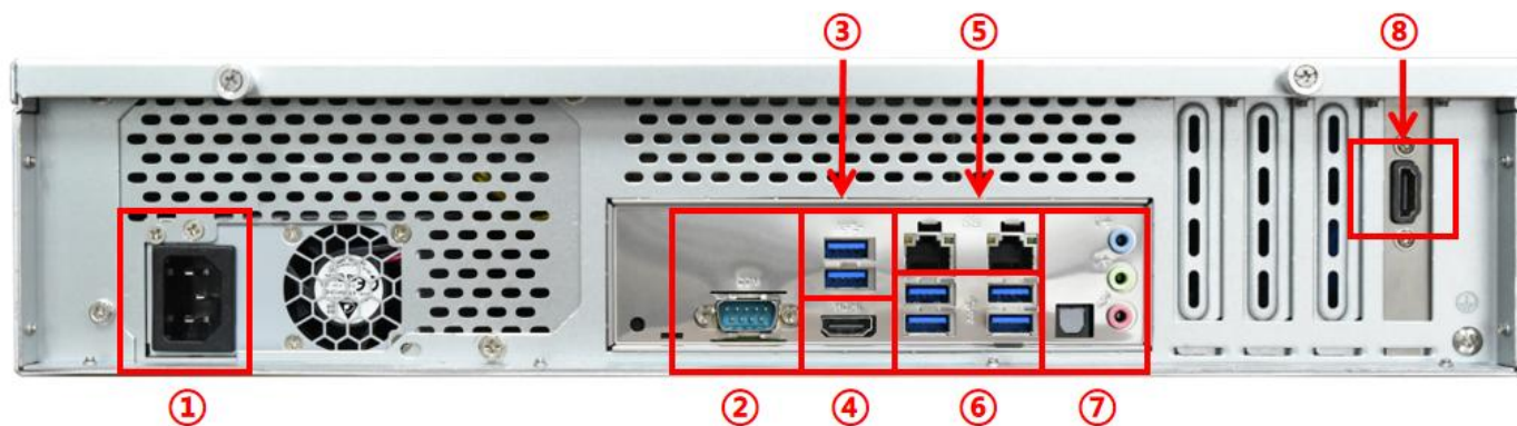
后面板
