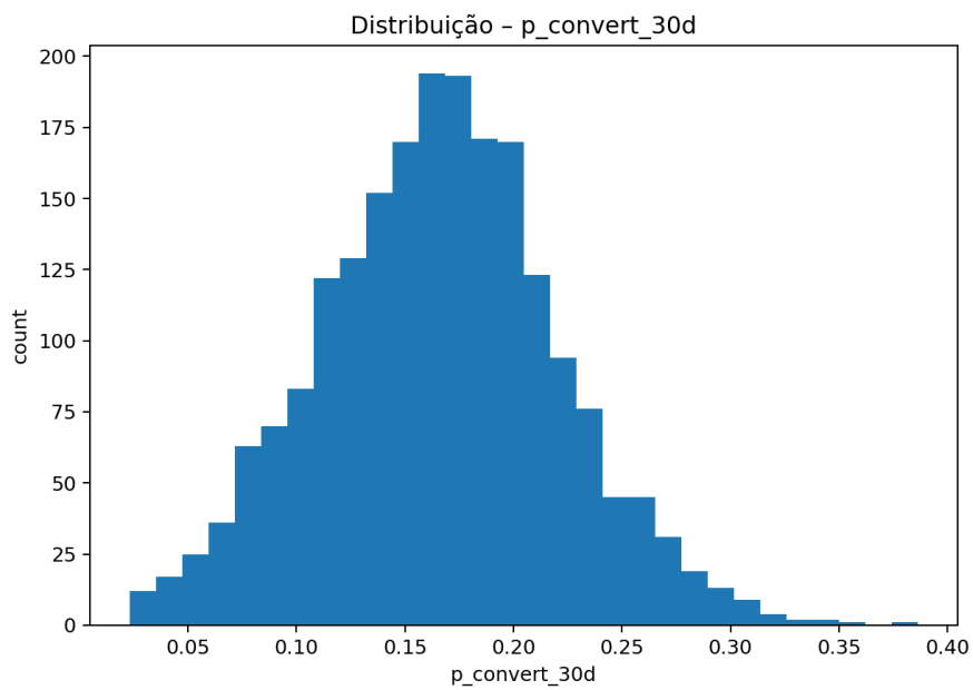
Distribuição - p_convert
