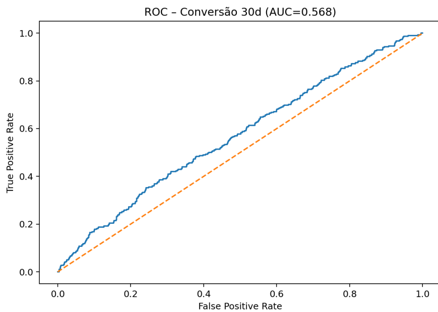
ROC – conversão
