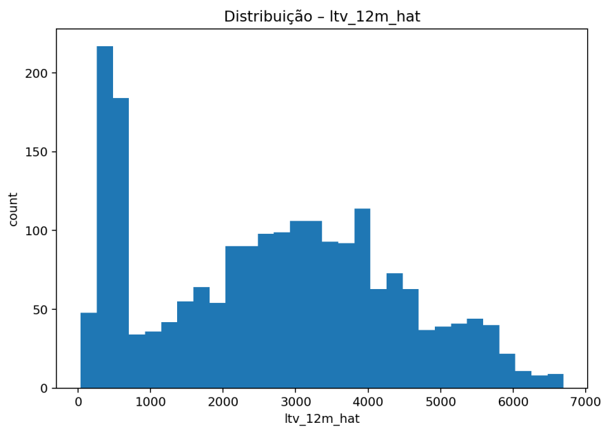
Distribuição – LTV_hat
