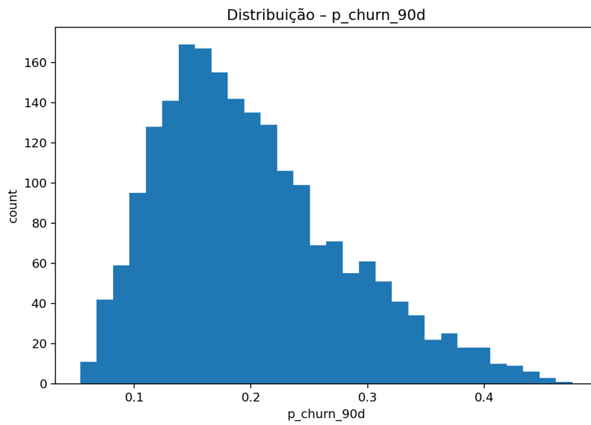
Distribuição - p_churn
