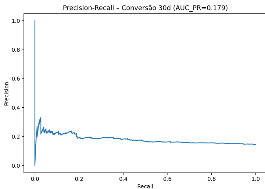
PR – conversão
