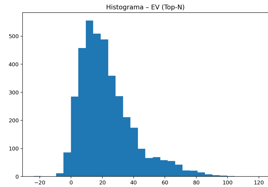
Histograma - EV
