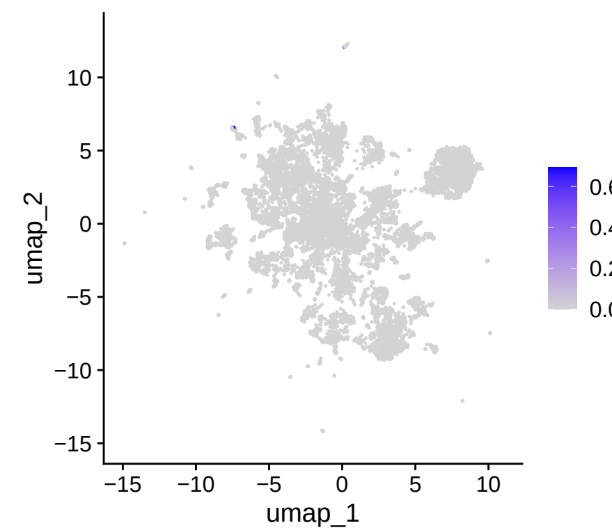
MME
