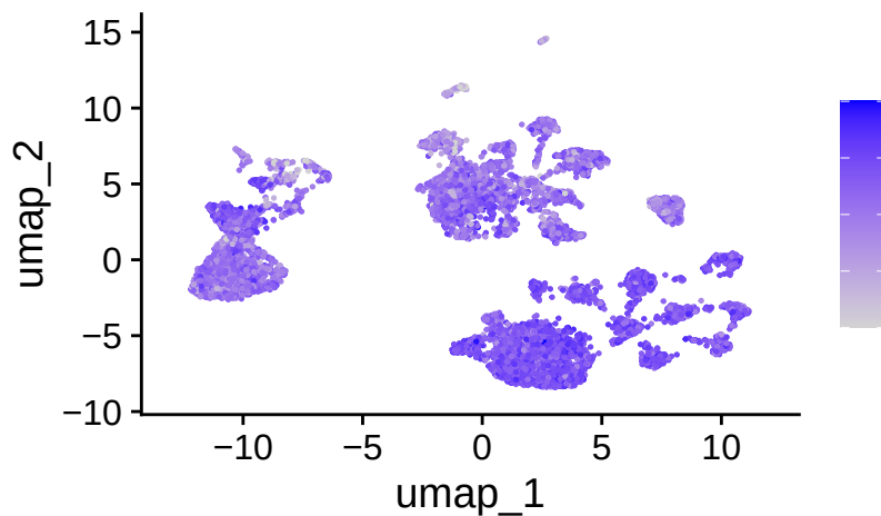
FLT3
