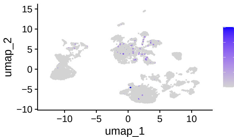
FLT3
