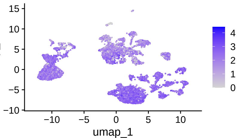
CD86
