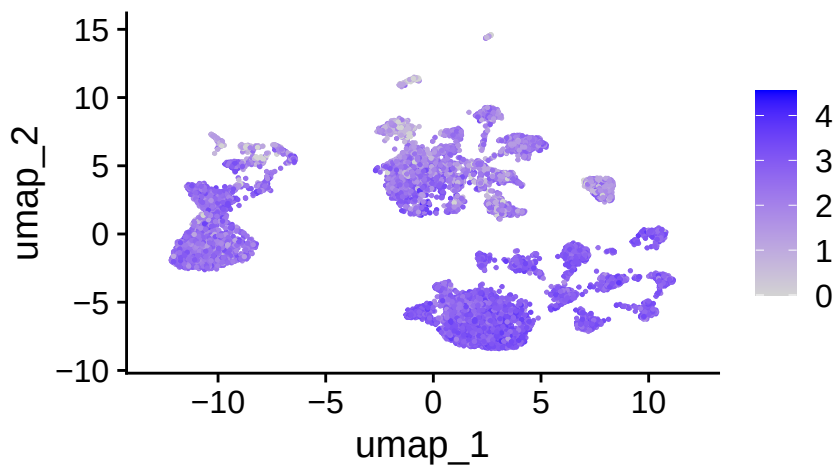
ITGAX
