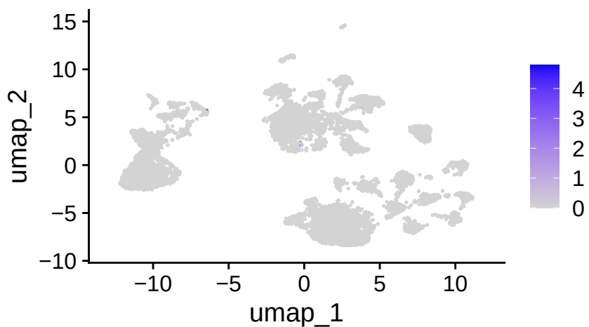
LYZ
