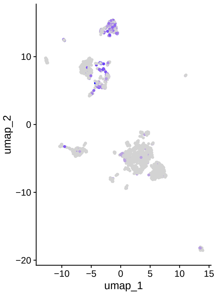
CD40
