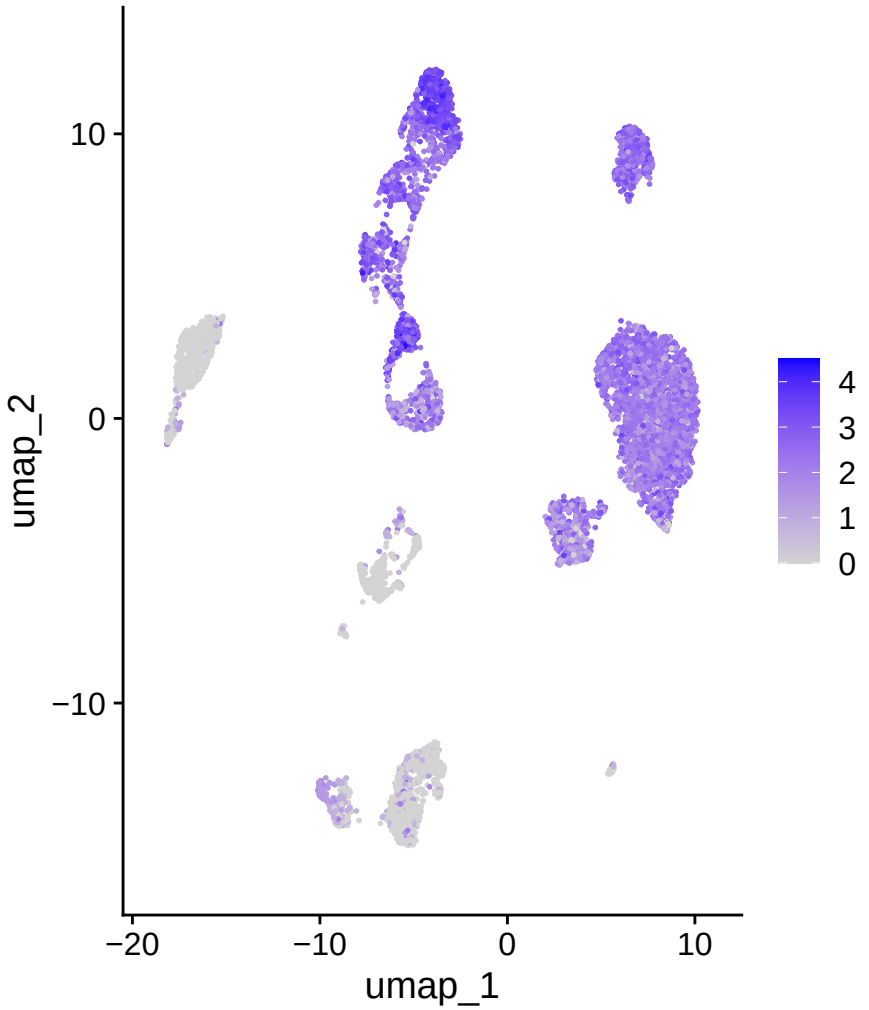
MS4A1
