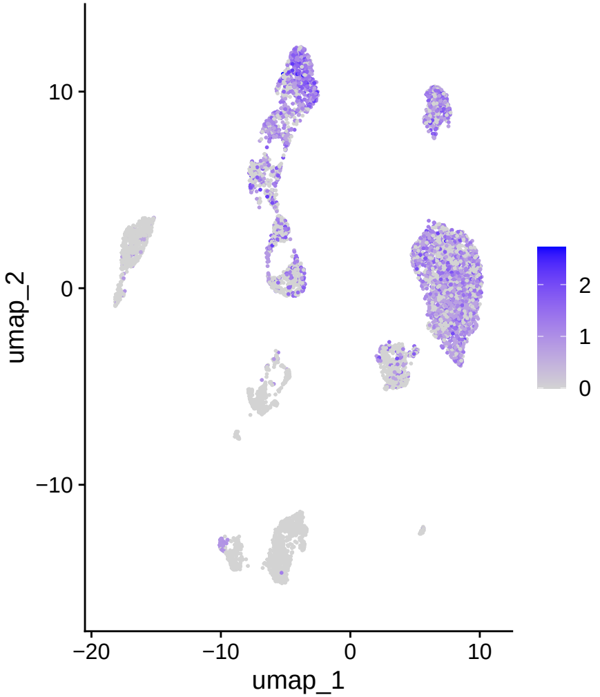
MS4A1
