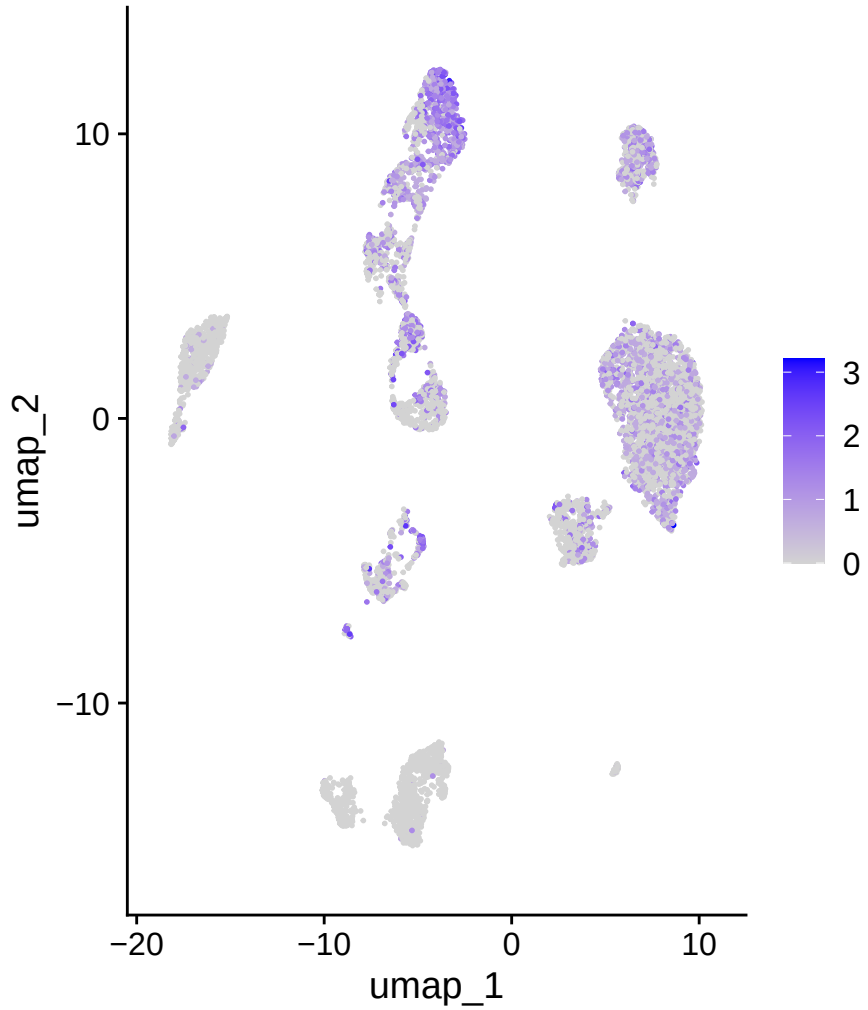
CD40
