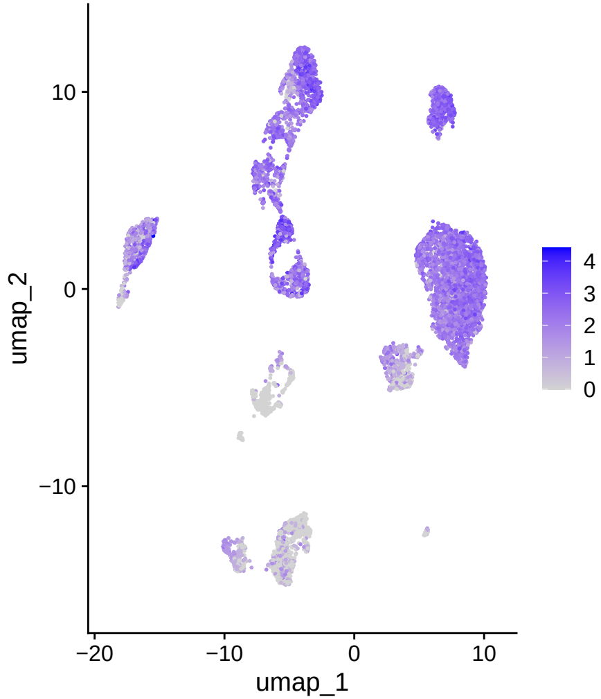
CD40
