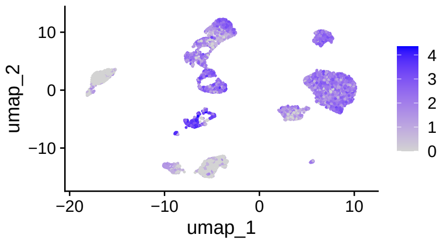
FLT3
