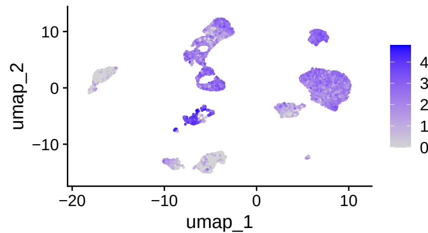
ITGAX
