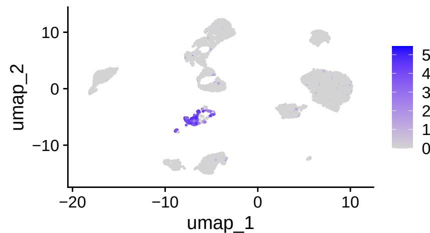
LYZ
