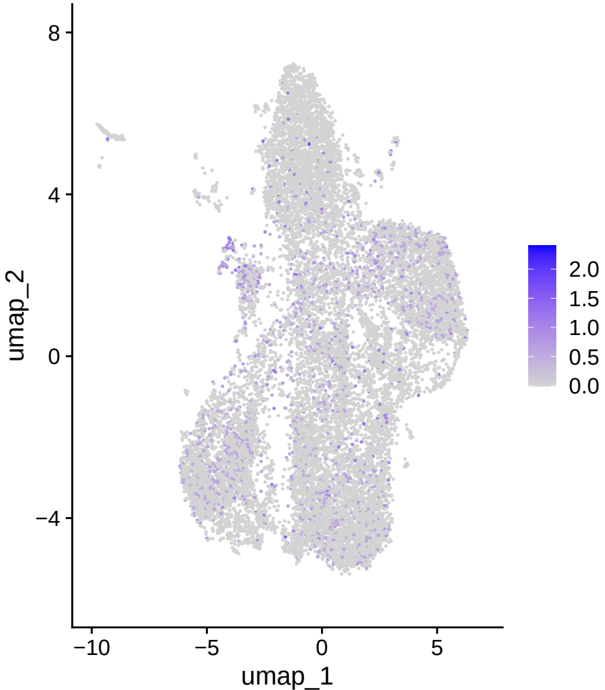
MS4A1
