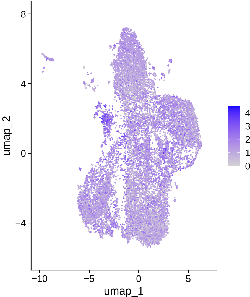
CD40
