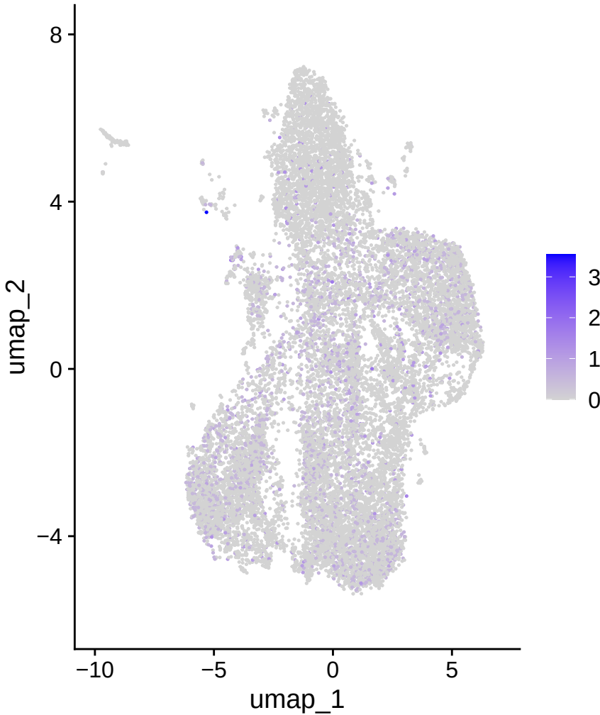
CD40
