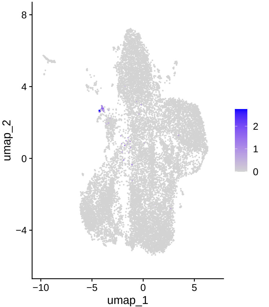
MS4A1
