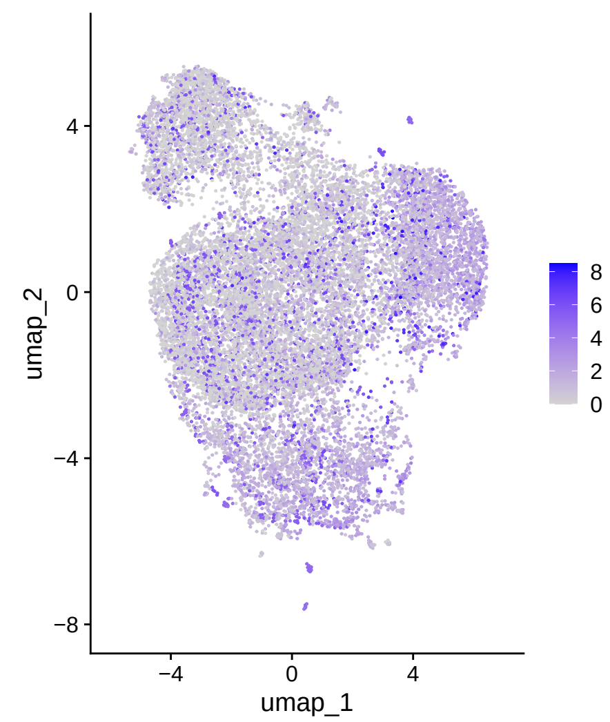
IGHG2
