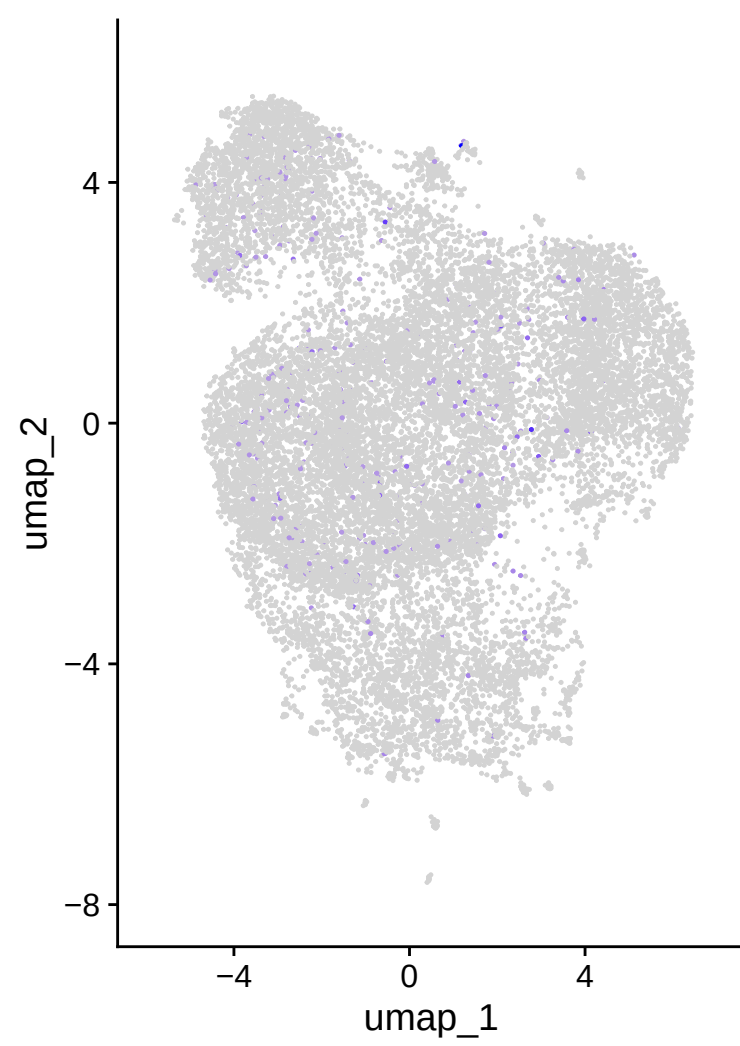
IGHG3
