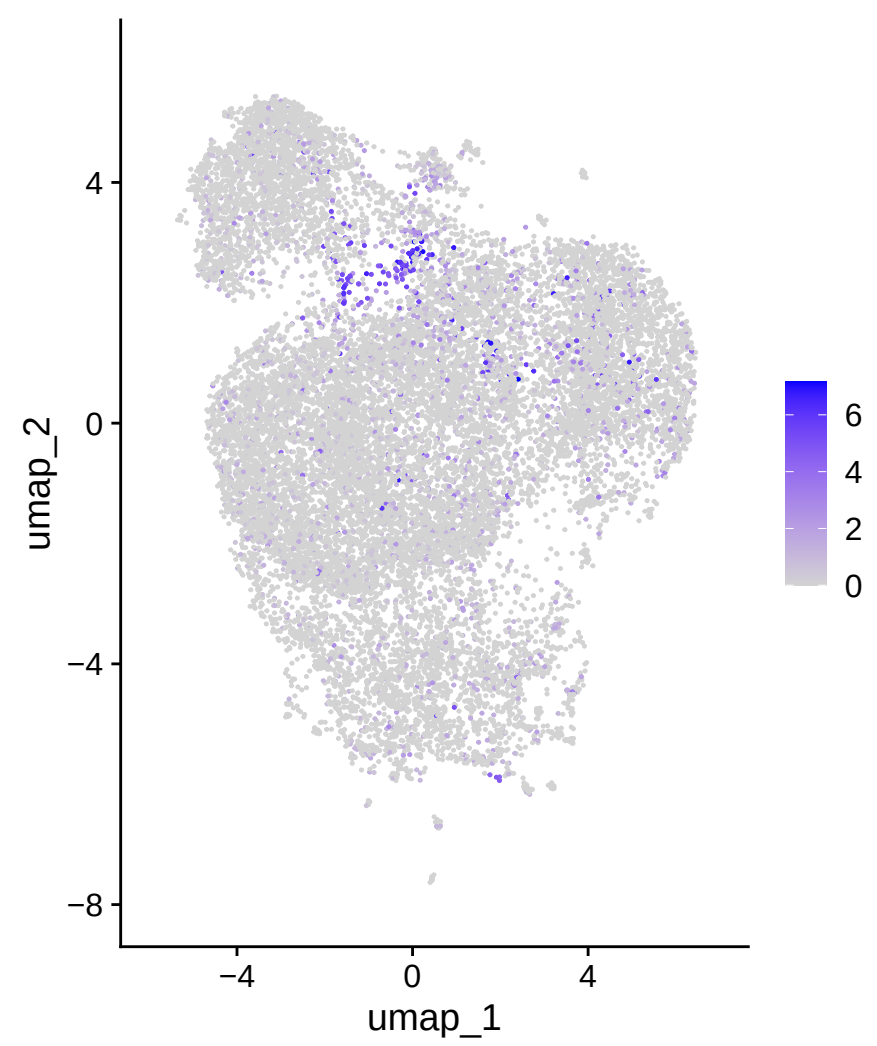
IGHG4
