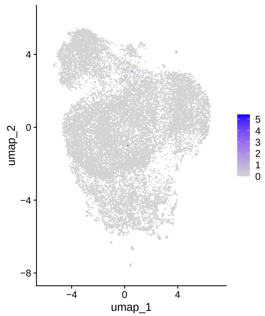
IGHE
