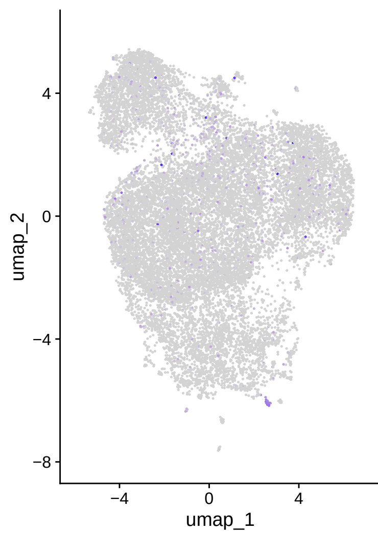
IGHA2
