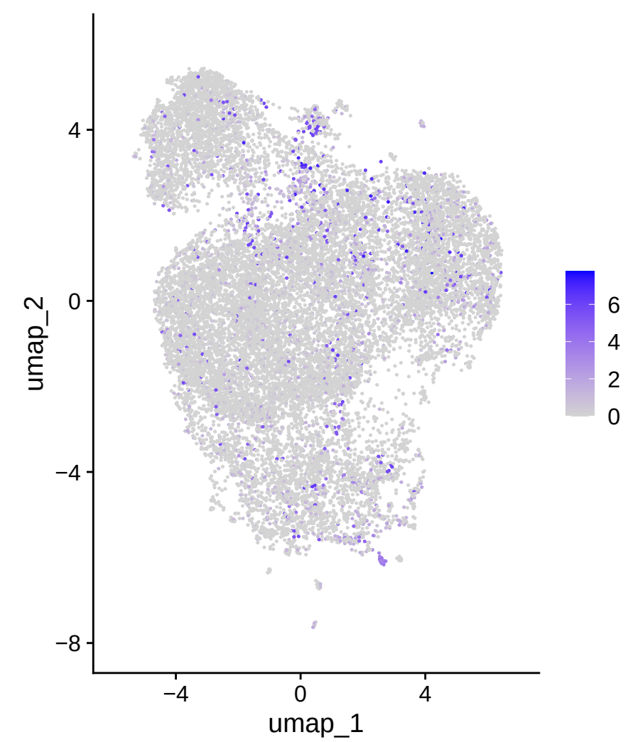
IGHA1
