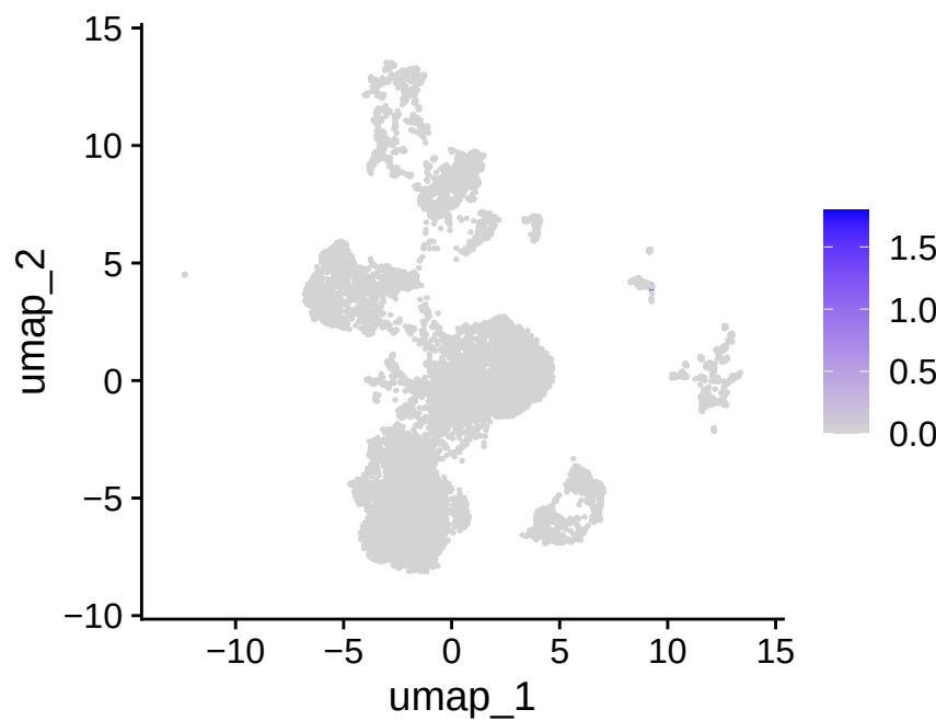
CD8A
