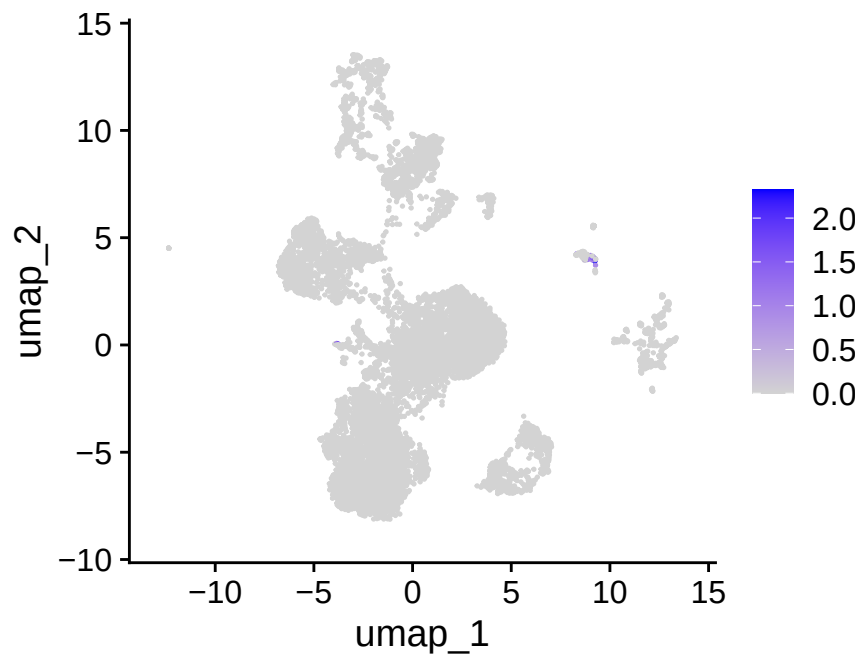
TRBC1
