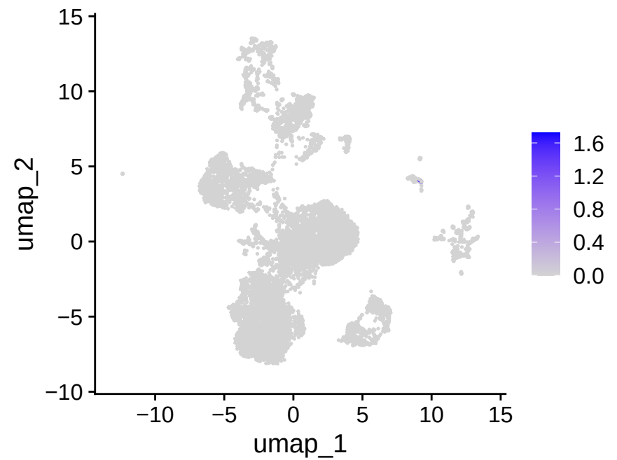
CD2
