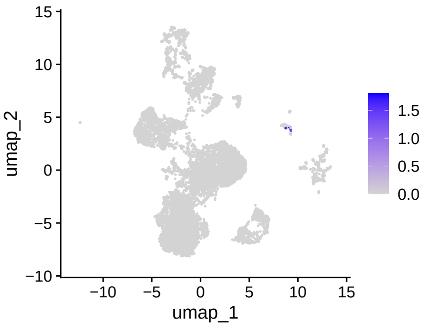
CD4
