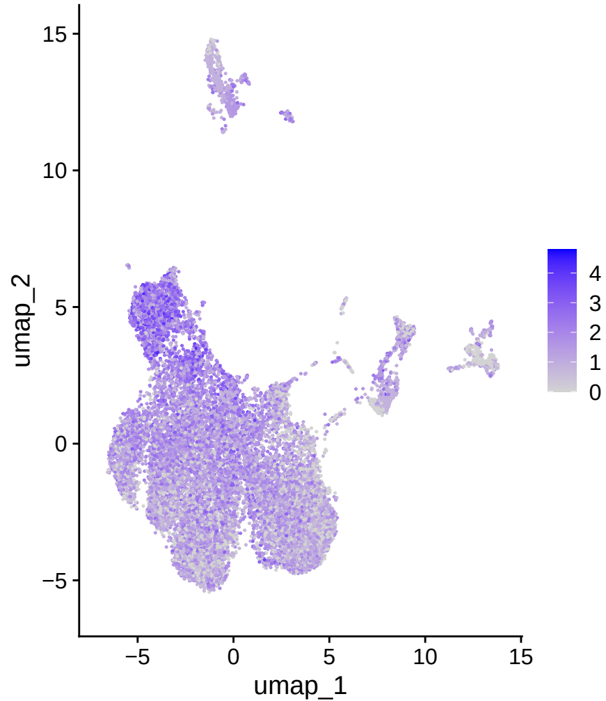
IRF4
