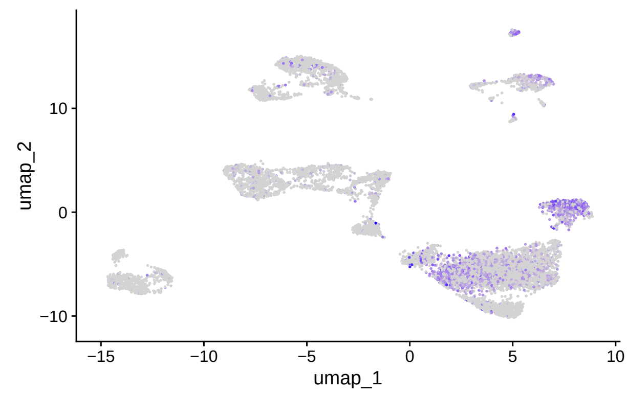
TXNIP
