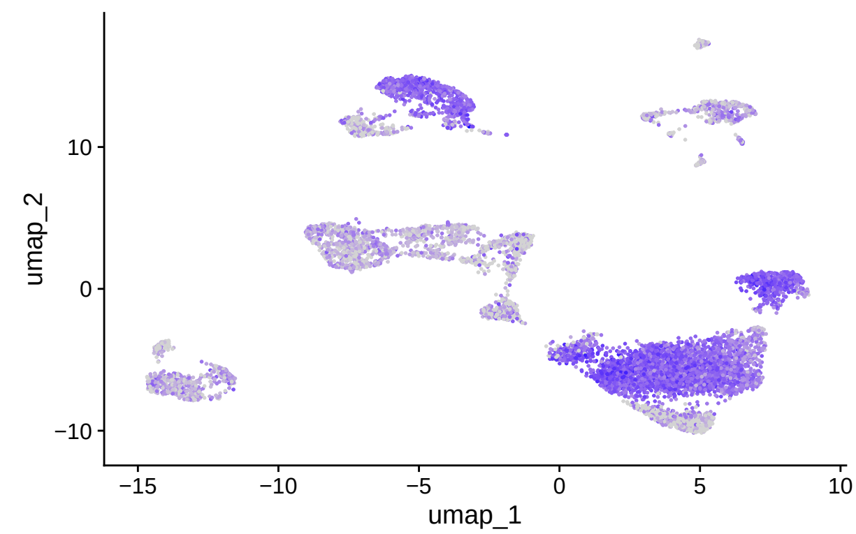
IL4R
