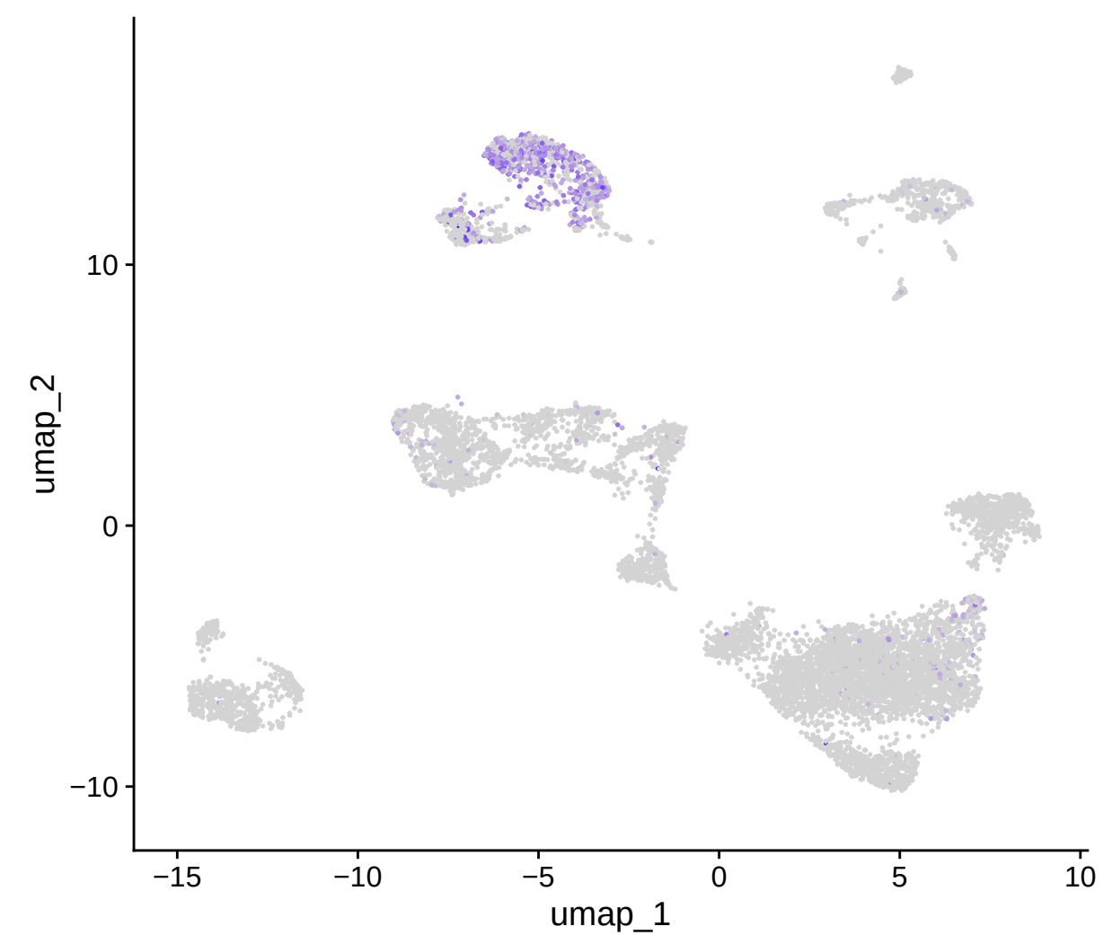
CD40LG
