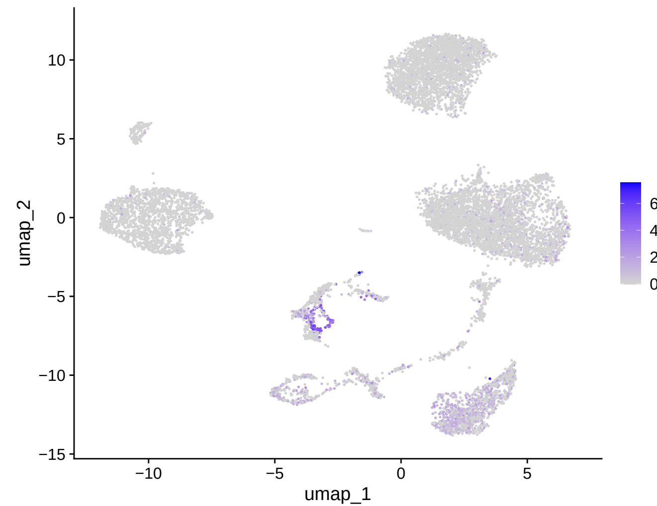
IGHG3
