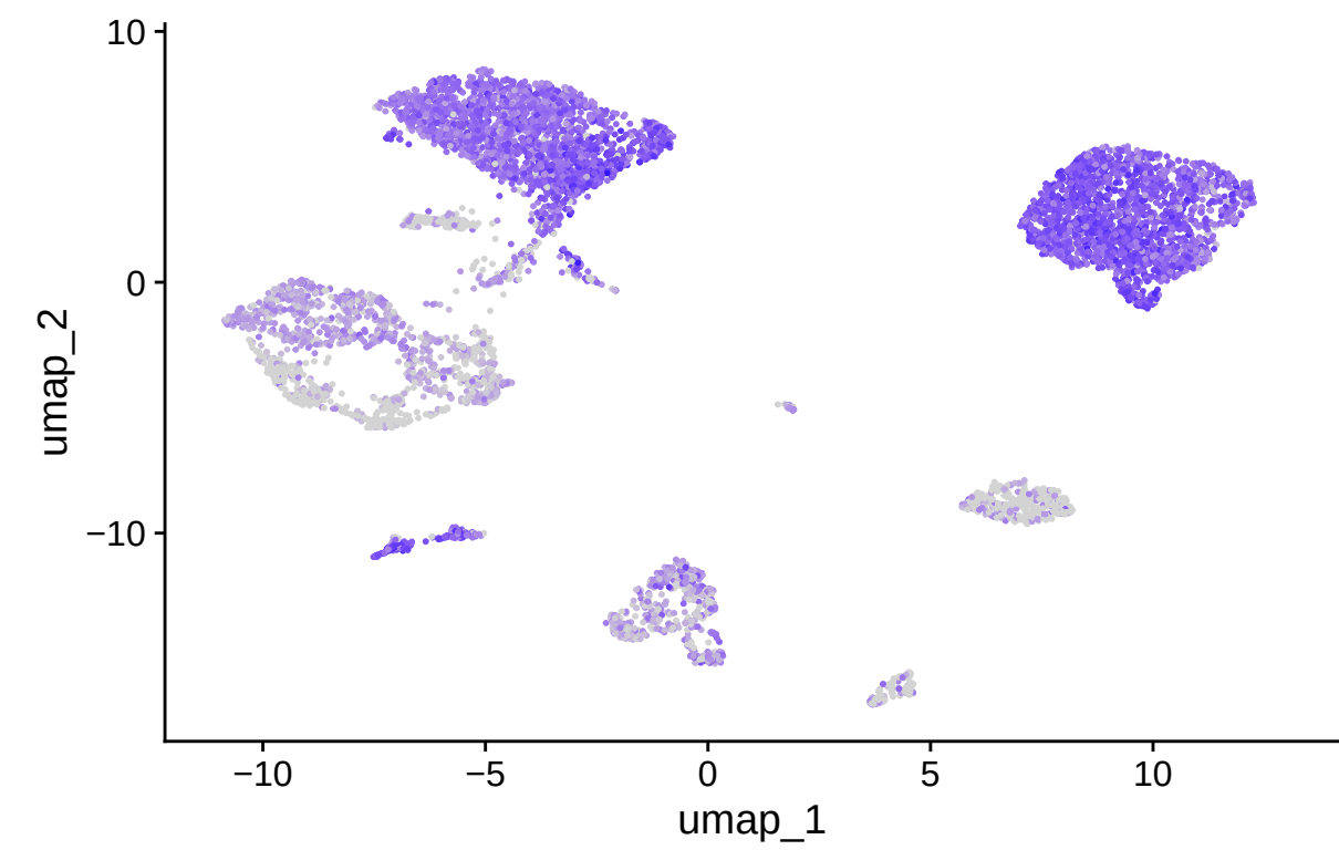
IL4R
