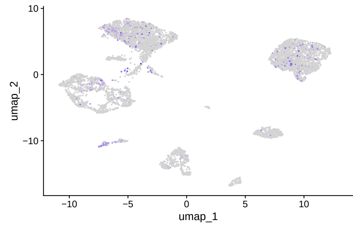
TXNIP
