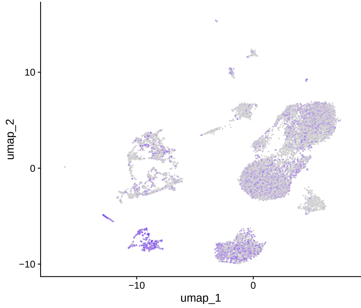
XBP1
