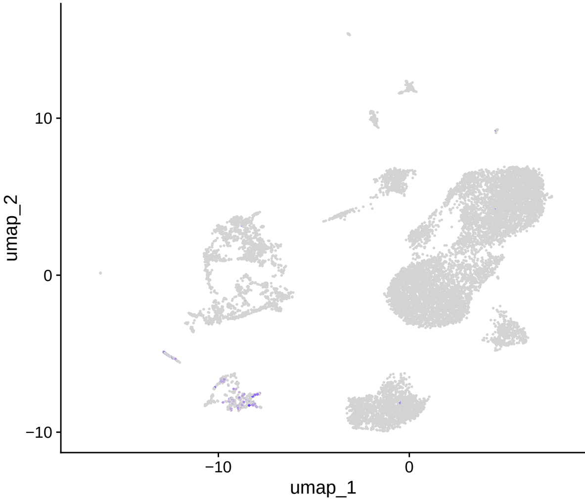
SDC1
