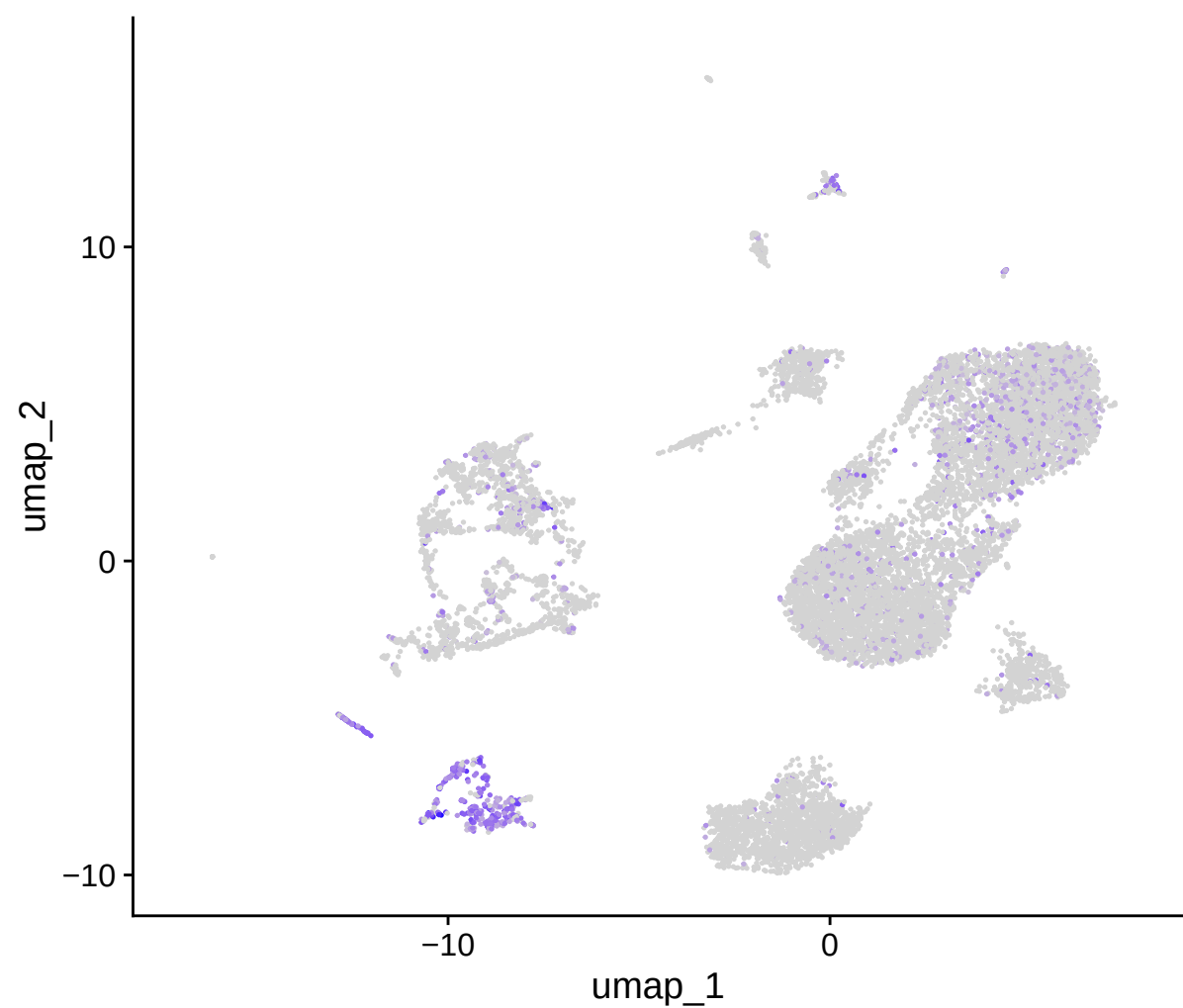
PRDM1
