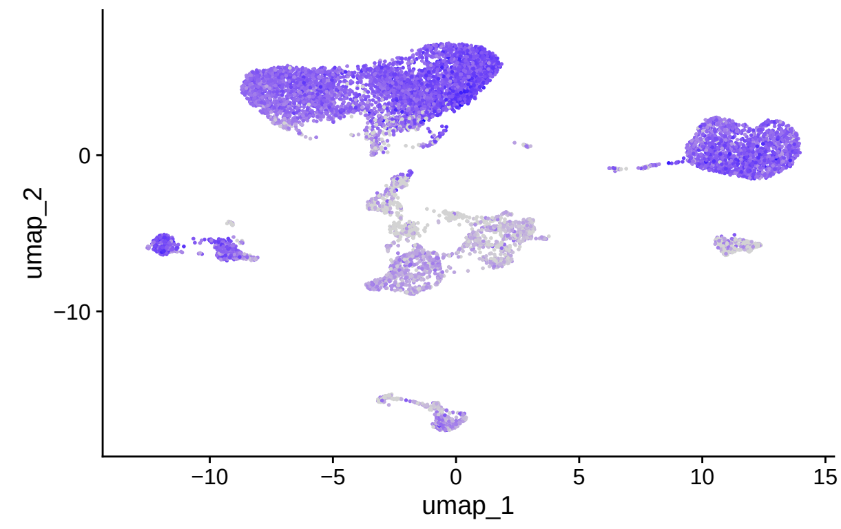
IL4R
