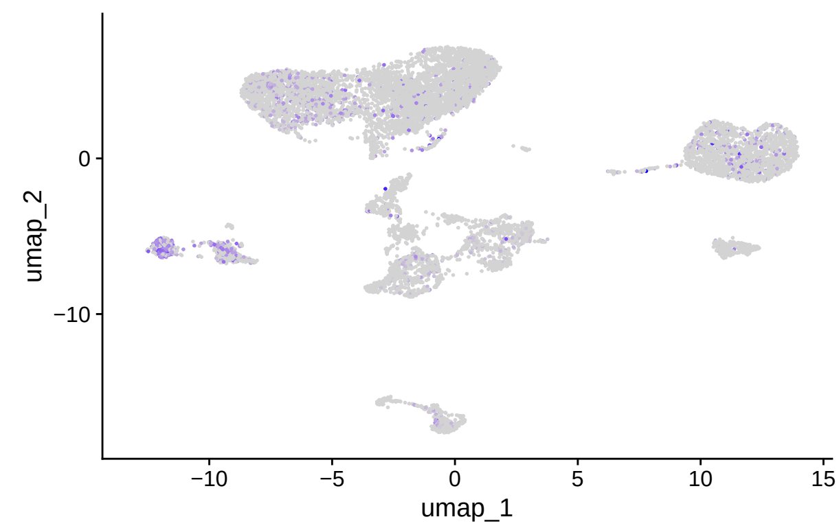
TXNIP
