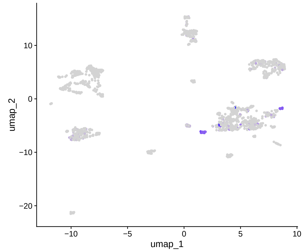
IGHG3
