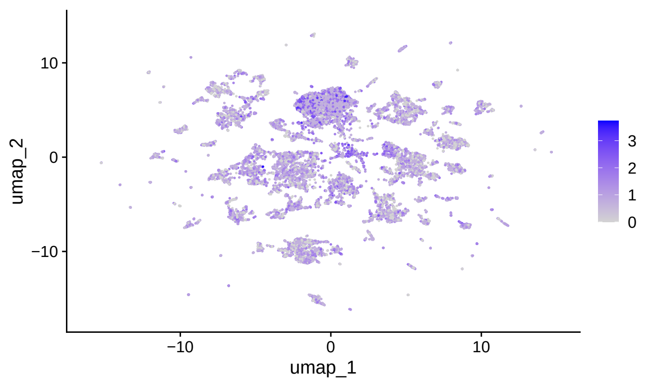
rna_SERPINA9
