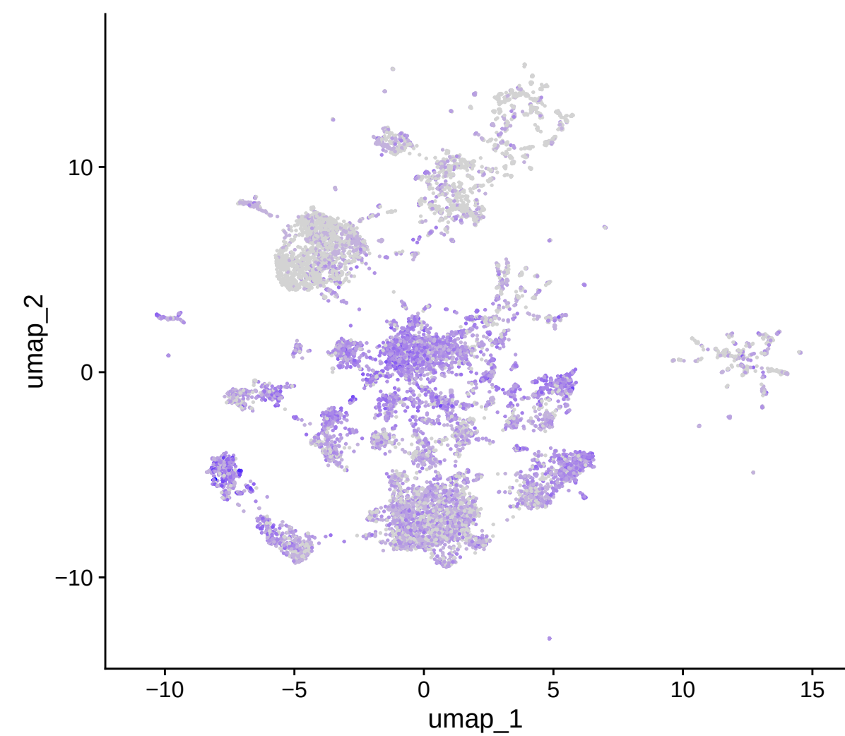
VIM
