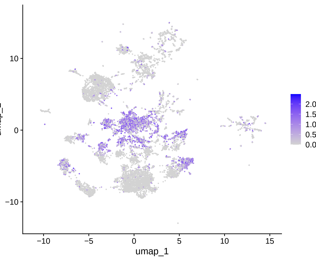
AIM2
