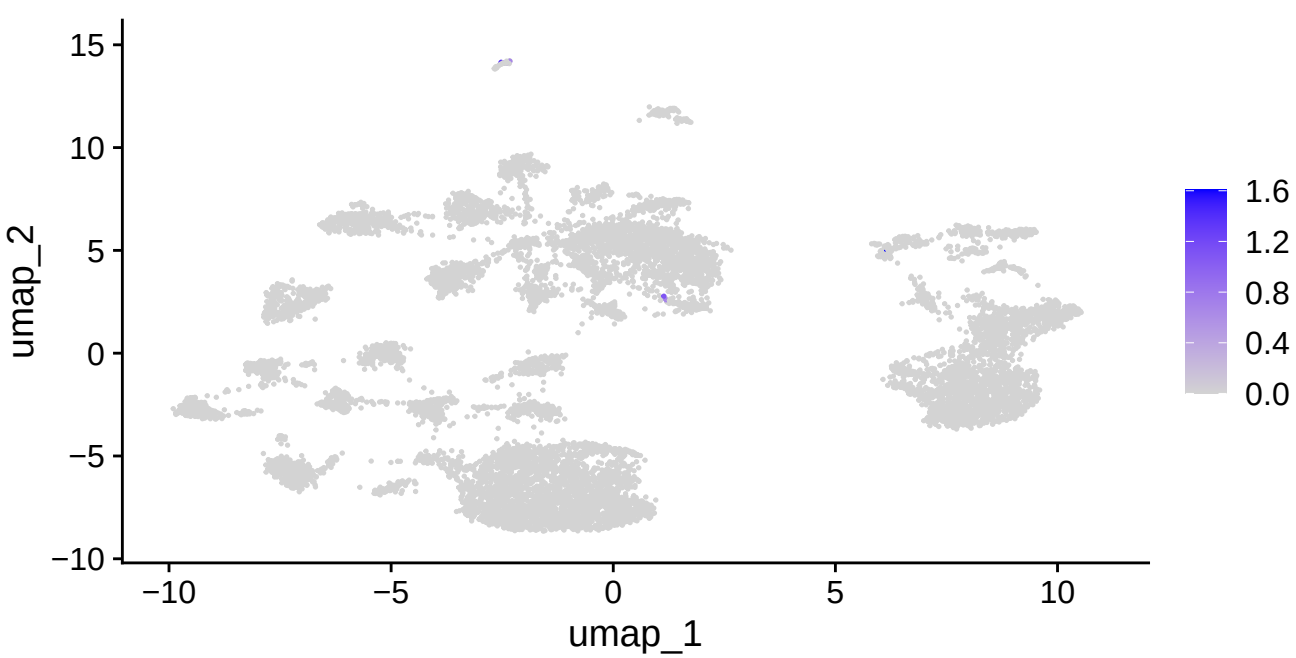
CD4
