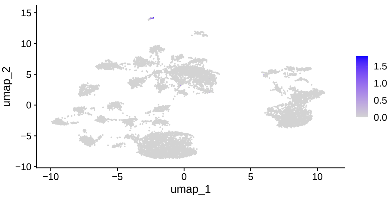
CD3E
