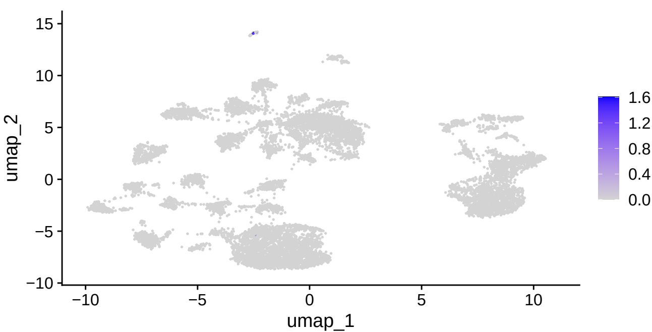
CD8A
