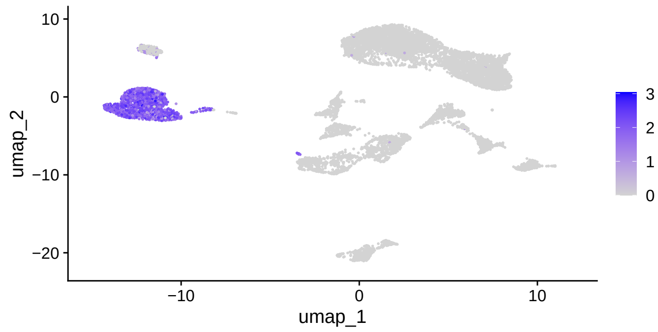
CD4
