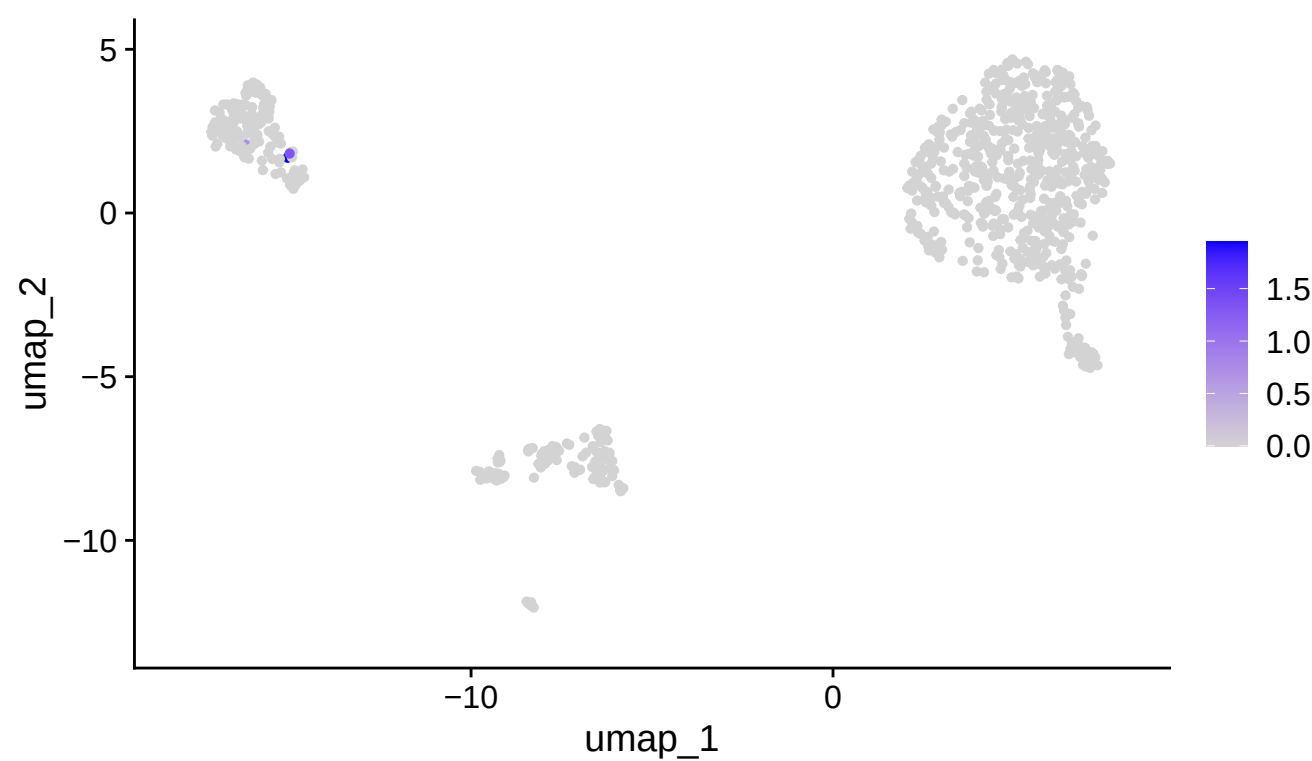
SERPINA9
