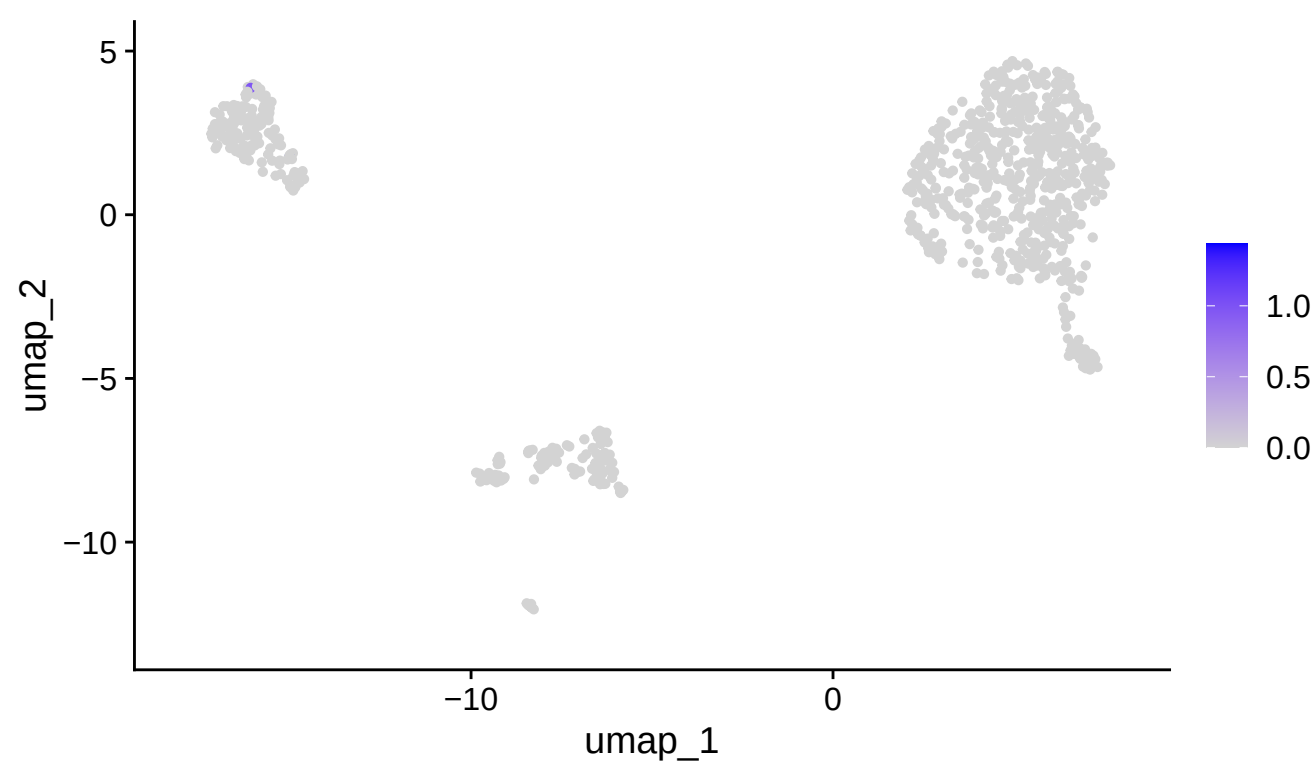
CD38
