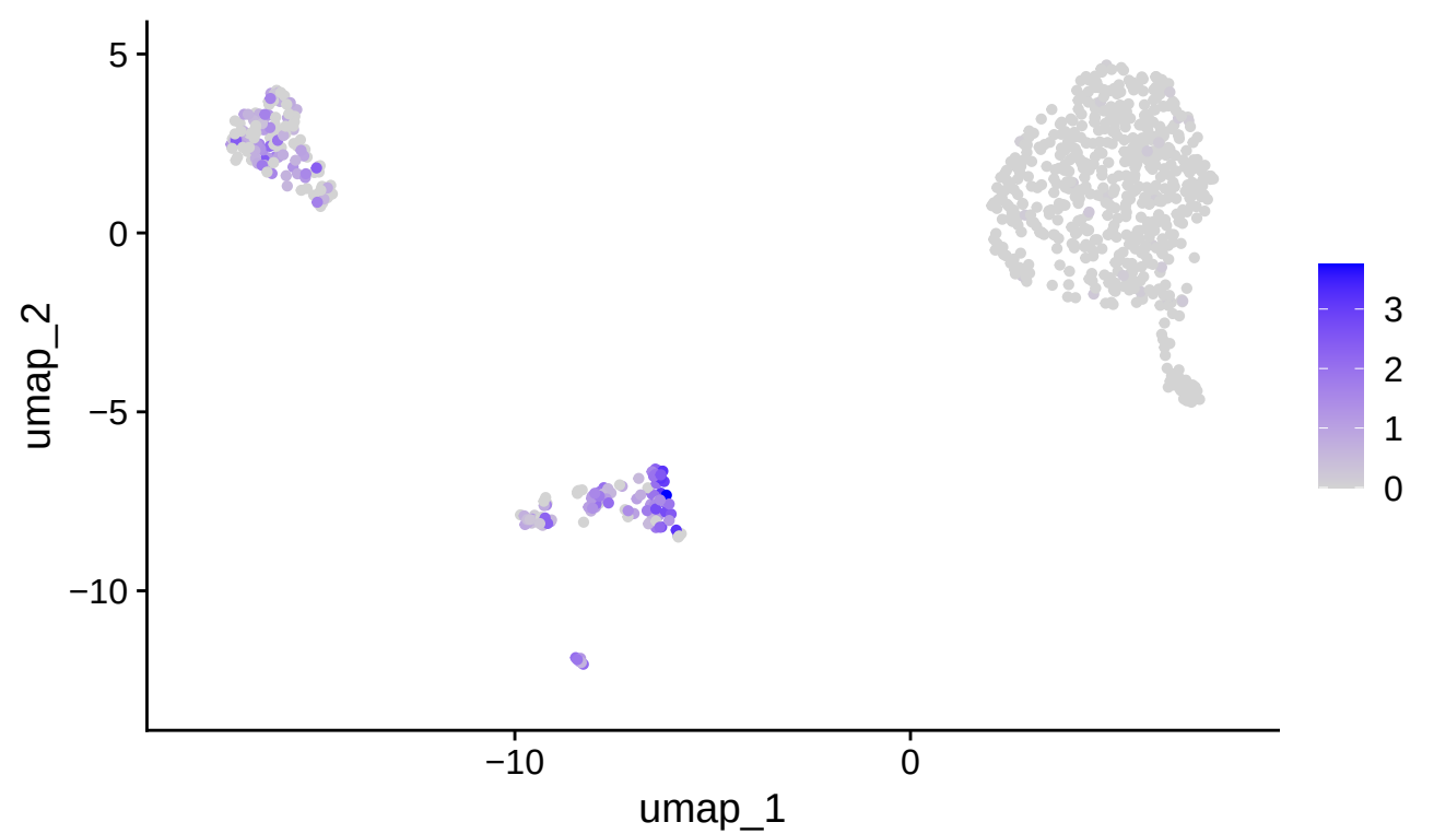
AICDA
