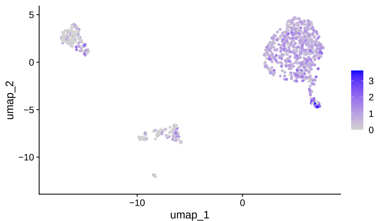
SERPINA9
