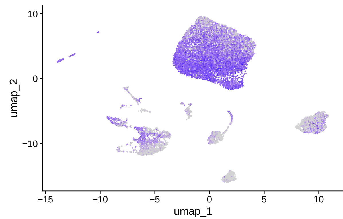
IL4R
