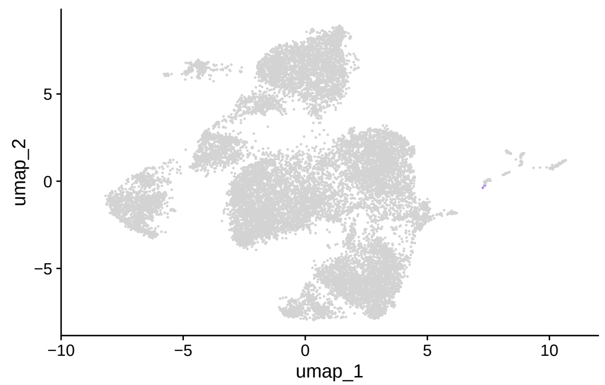
CD38
