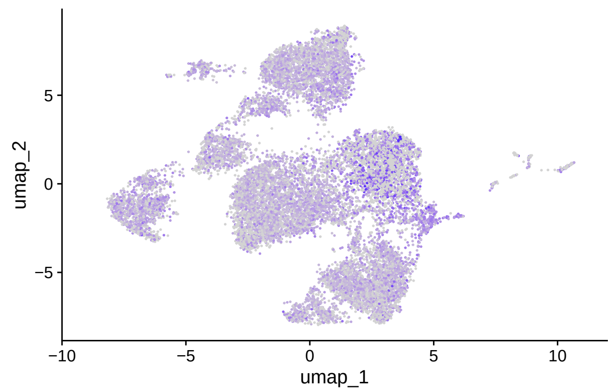
SERPINA9
