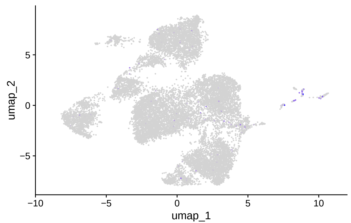
AICDA
